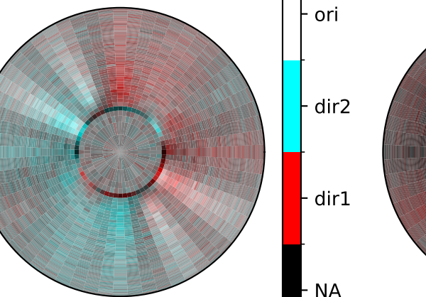
neuron 4
