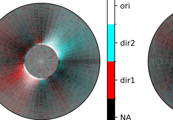
neuron 5
