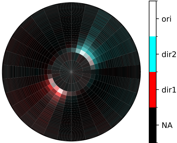
neuron 5
