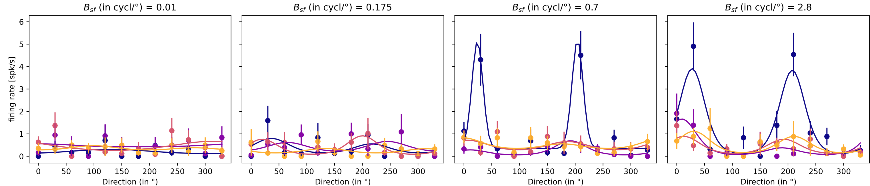
neuron 15
