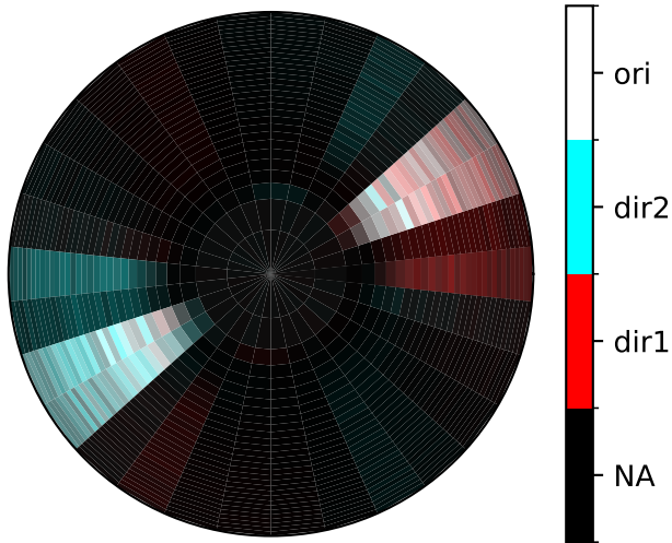
neuron 15
