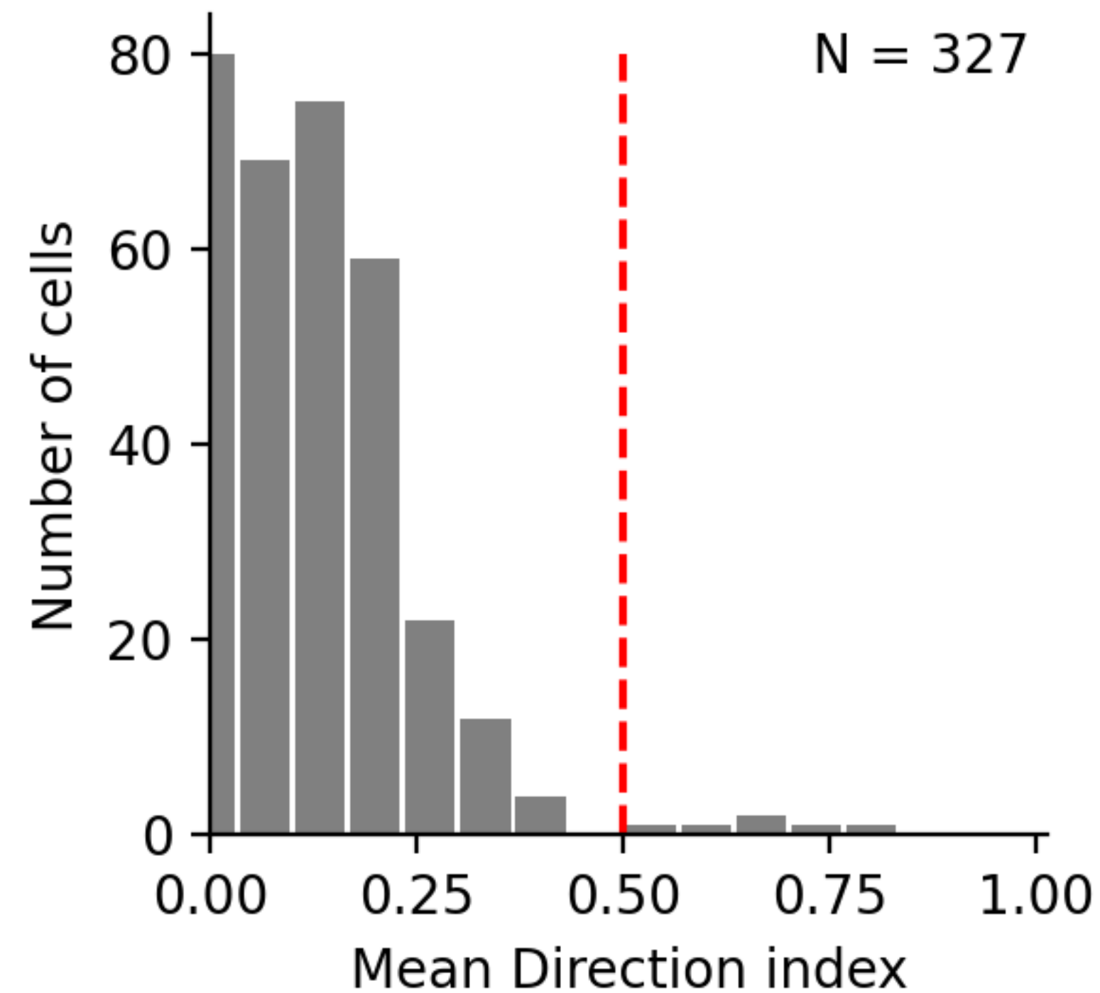
6 neurons Dir Selec
