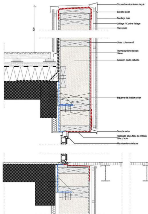
Détail : Coupe de principe dans la façade coté balcons
