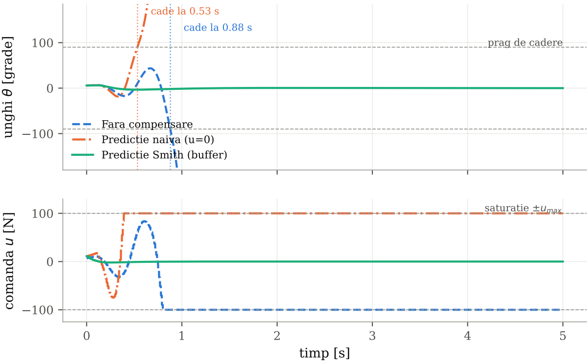
Ablatia compensarii latentei, \tau = 100 ms, LQR la 100 Hz
