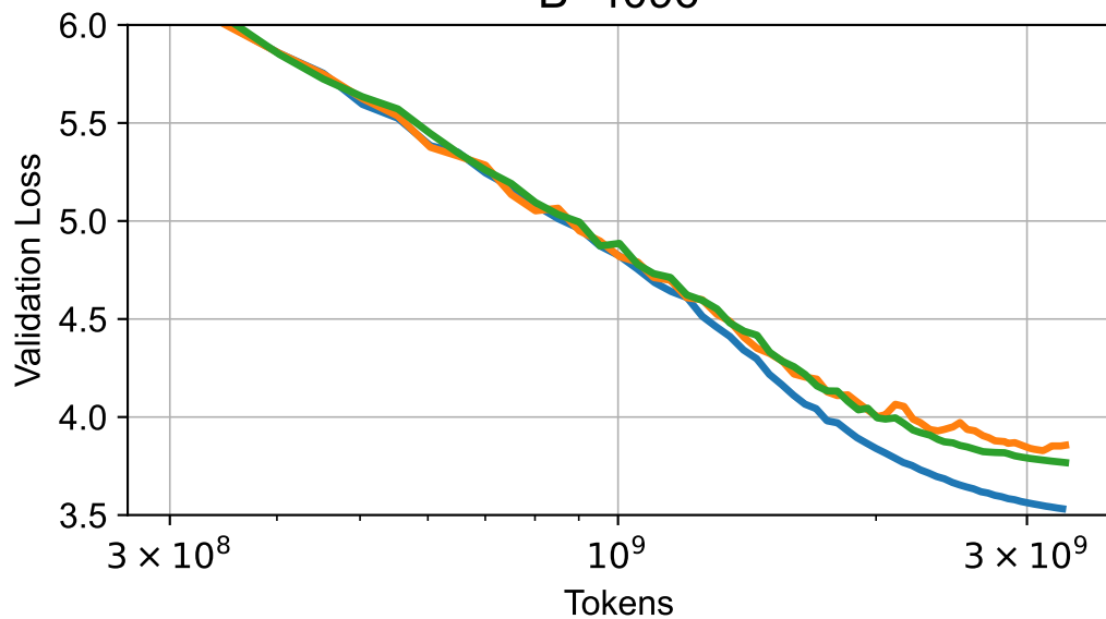
B=4096
