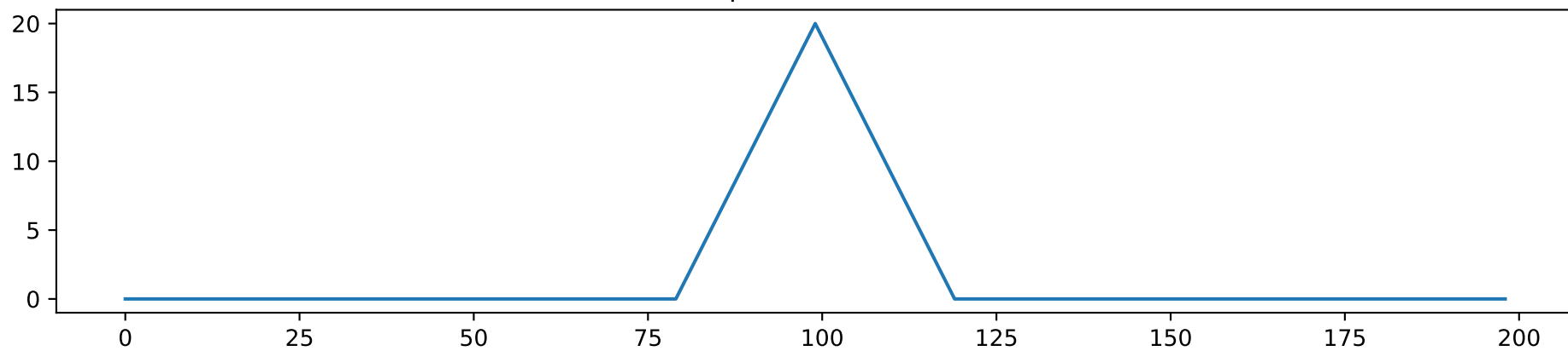
Dupa 2 convolutii
