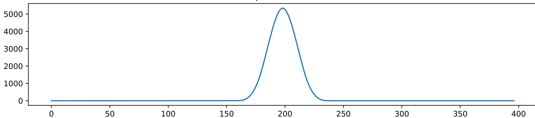
Dupa 3 convolutii
