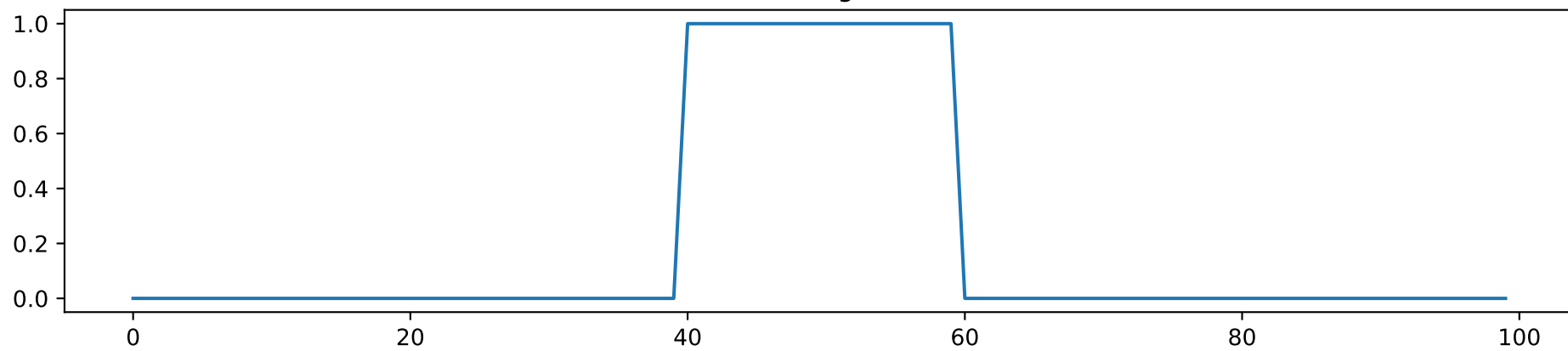
Dupa 1 convolutie
