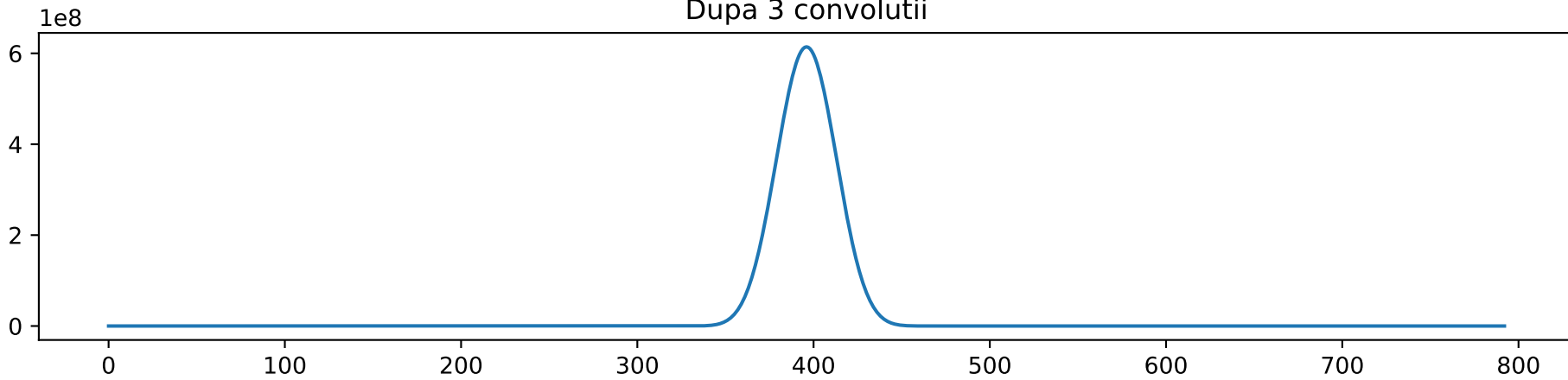
Dupa 3 convolutii
