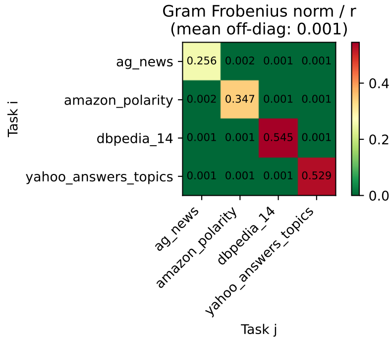
olora — task-pair similarity (A matrices)
