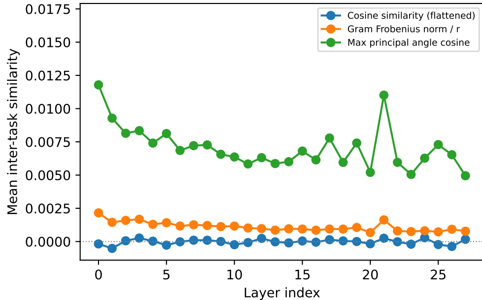
q_proj
