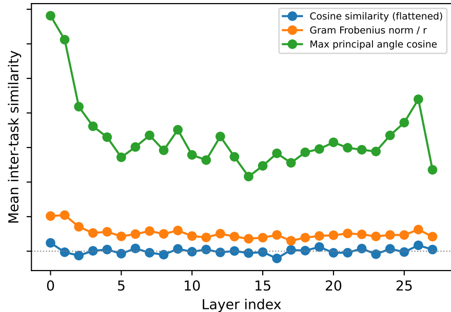
v_proj
