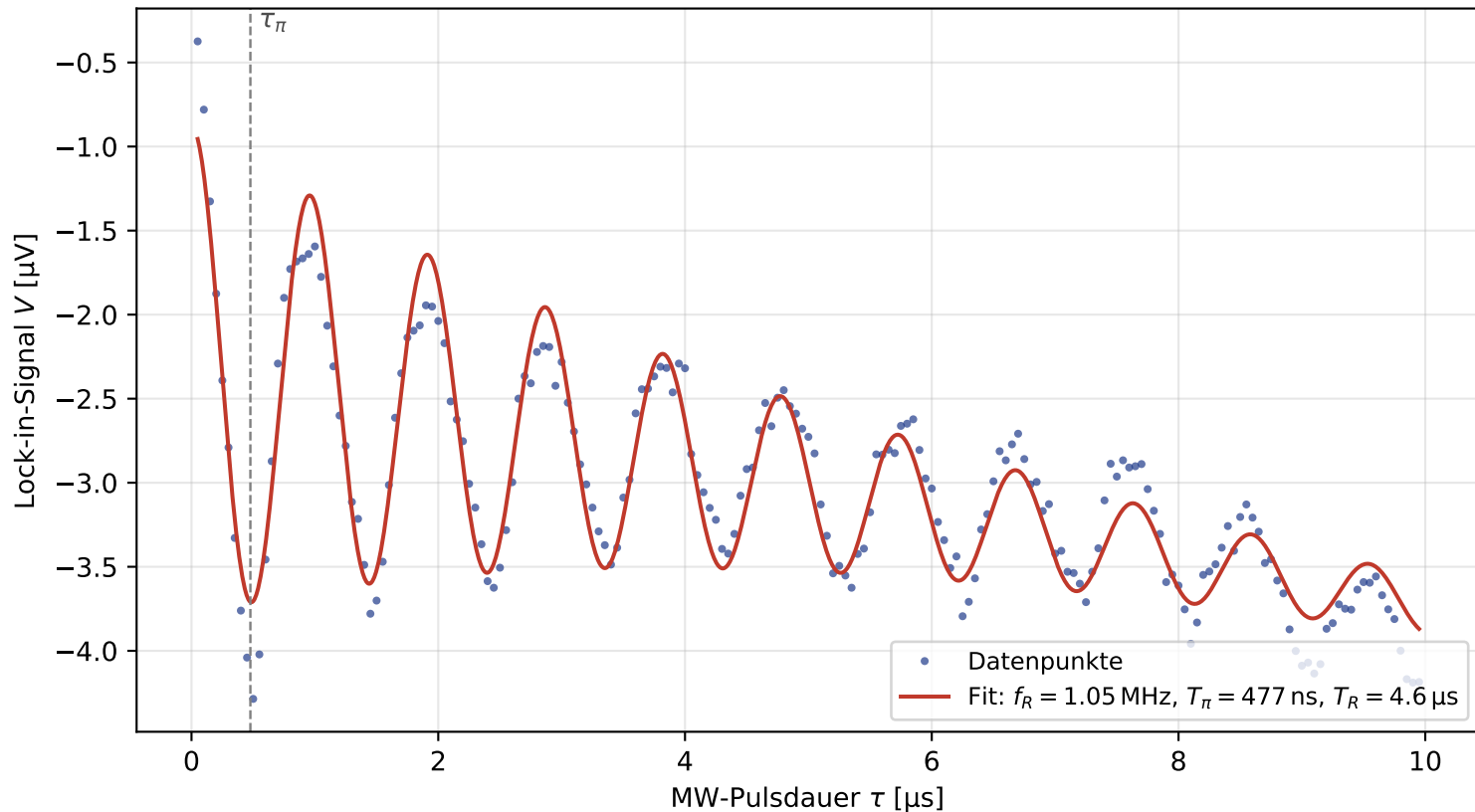
Rabi-Oszillation bei P_{\text{MW}} = 0 dB, f_{\text{MW}} = 2,7825 GHz
