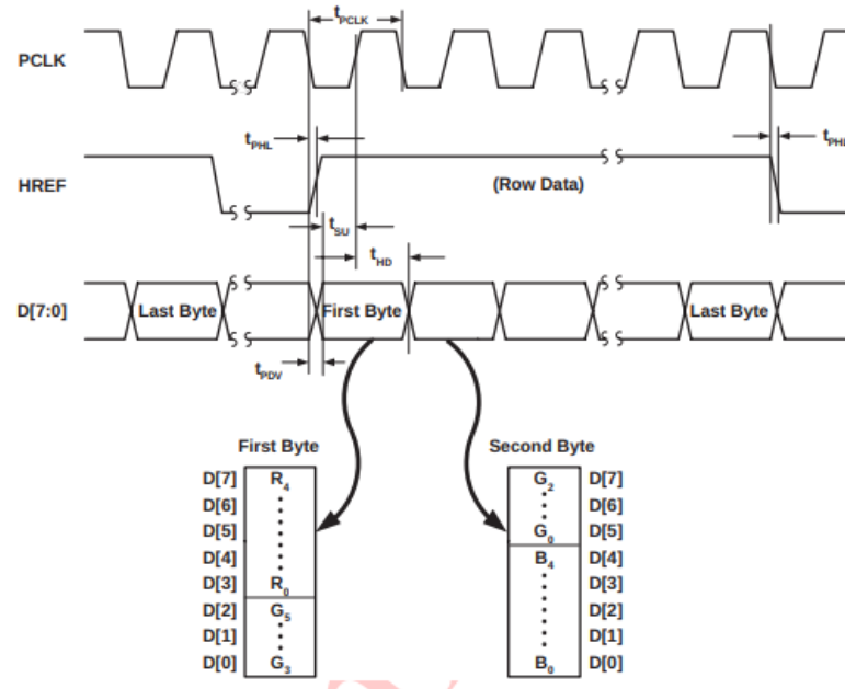
Gambar 3.2: Timing keluaran data RGB565 pada kamera OV7670
