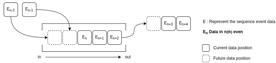
Gambar 2.4: Ilustrasi FIFO
