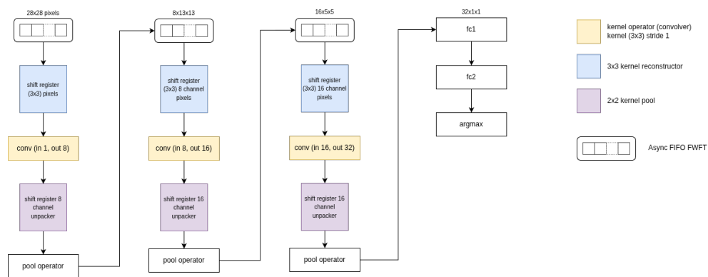
Gambar 4.8: Desain CNN Accelerator pada FPGA
