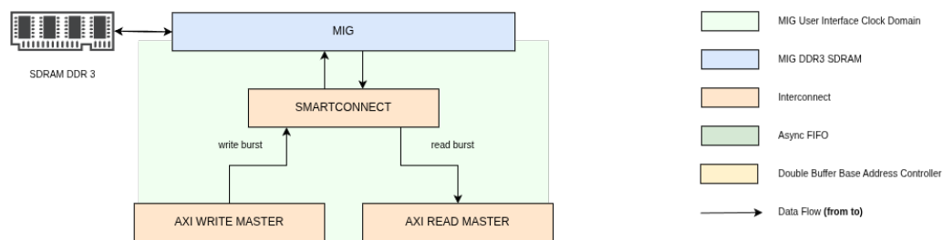
Gambar 2.7: Ilustrasi hubungan AXI, MIG, dan DDR pada sistem pemindahan data berbasis memori eksternal.
