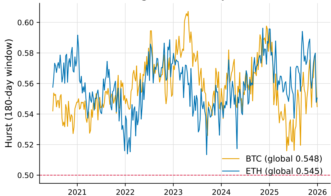
Rolling R/S Hurst exponent
