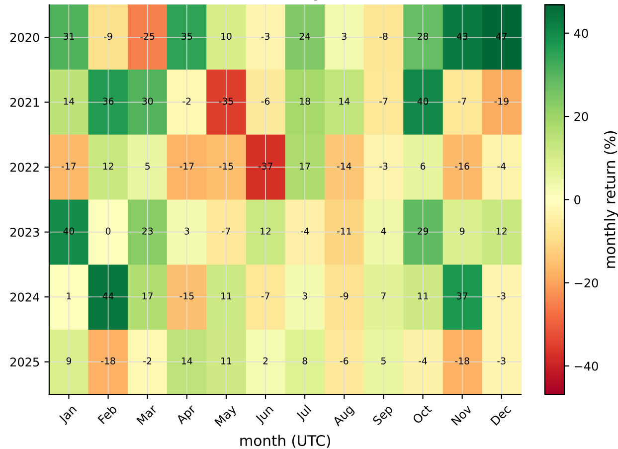
BTCUSDT - monthly return (%)
