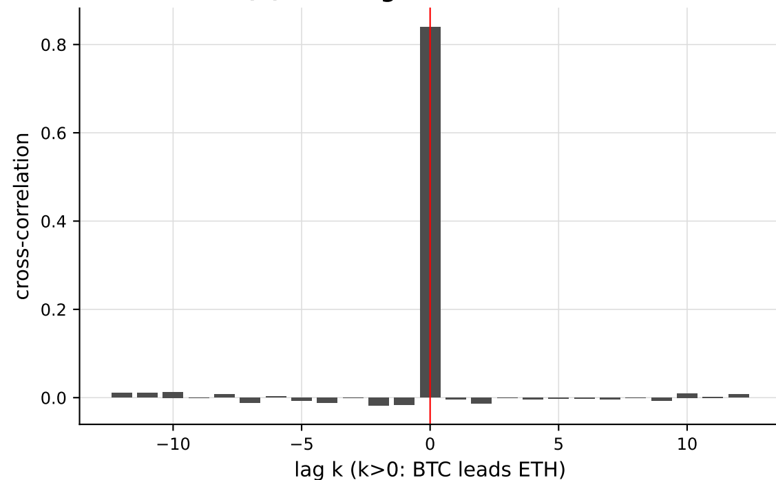
(d) Lead-lag cross-correlation
