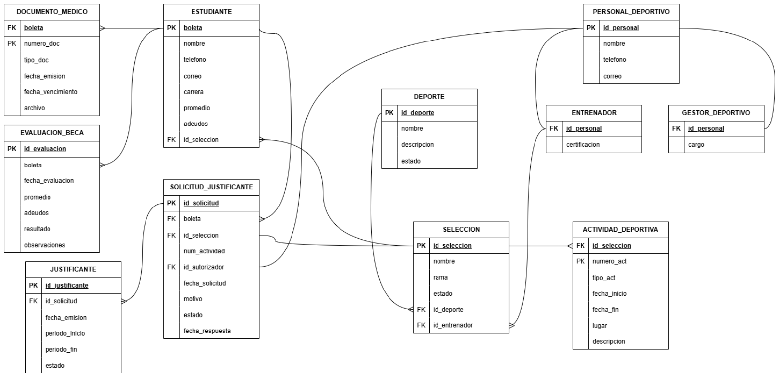
Diagrama en modelo de Crows feet
