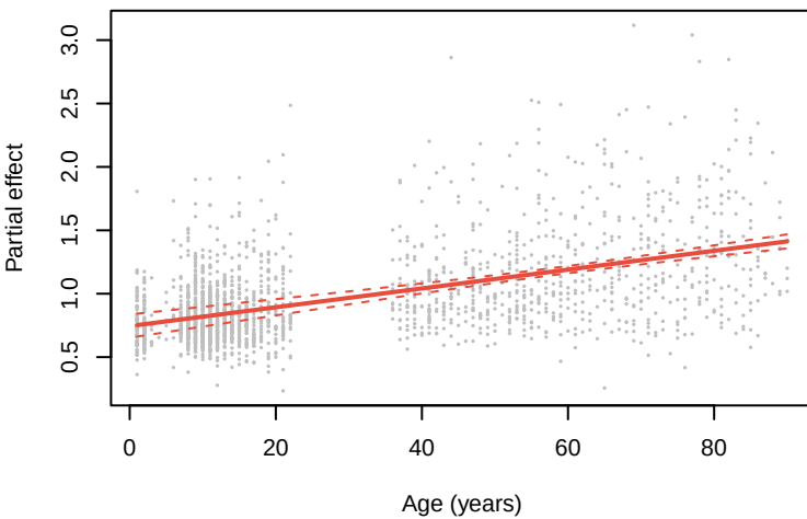
R23 | edf=1.0 | q=0.000
