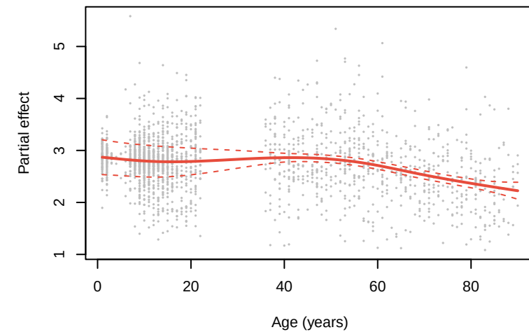
R16 | edf=3.3 | q=0.000
