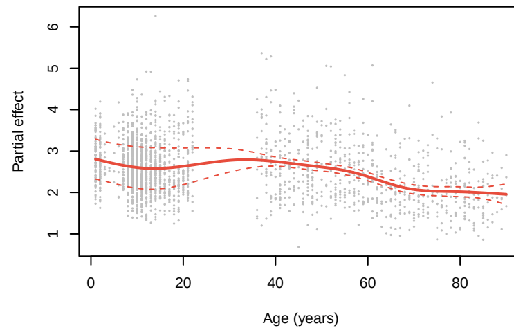
R26 | edf=1.0 | q=0.000
