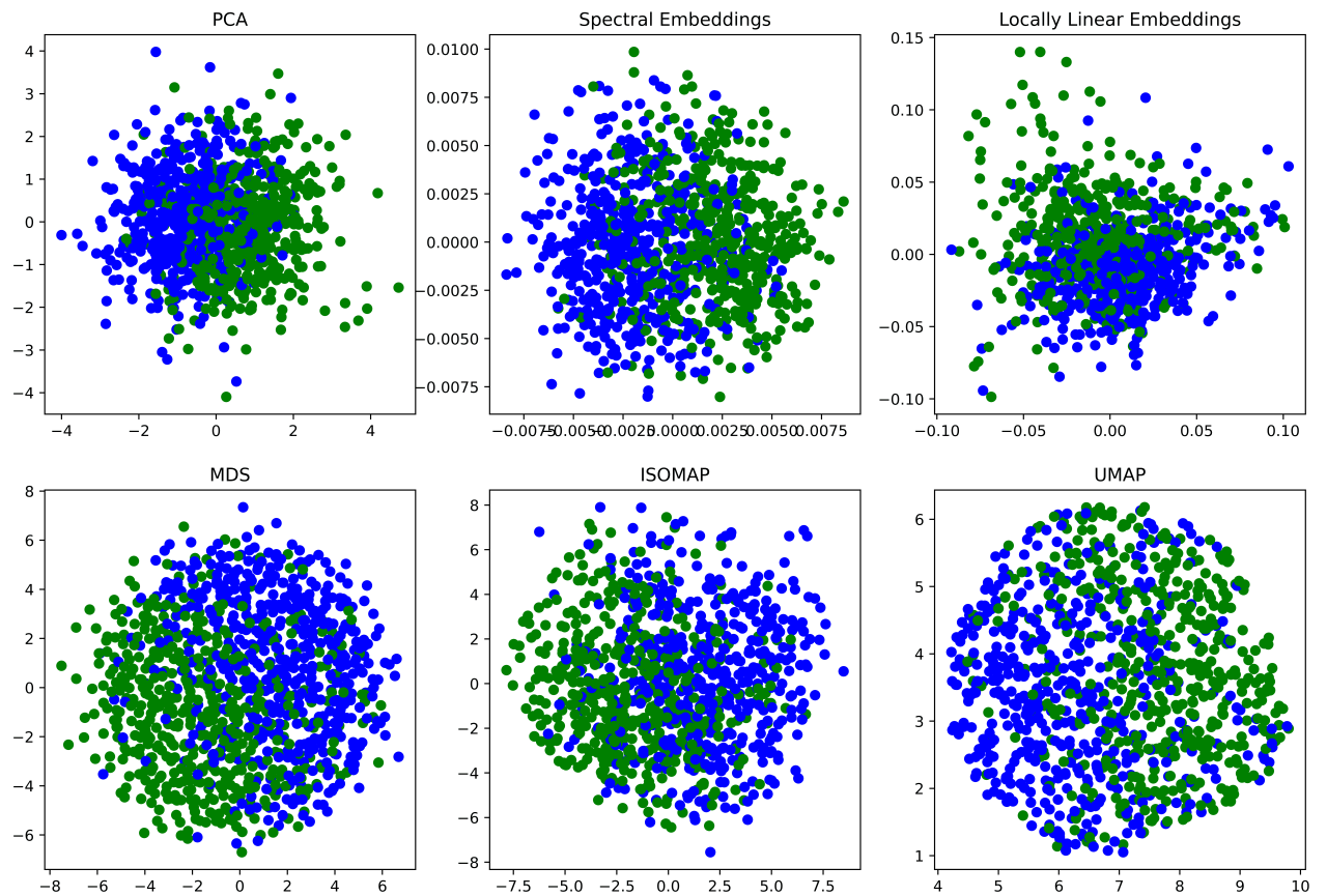
Рис. 5: Визуализация синтетических данных с параметром t = 0.8 после снижения размерности с 20 до 2 с использованием PCA, Spectral Embeddings, Locally Linear Embeddings, MDS, ISOMAP, UMAP.
