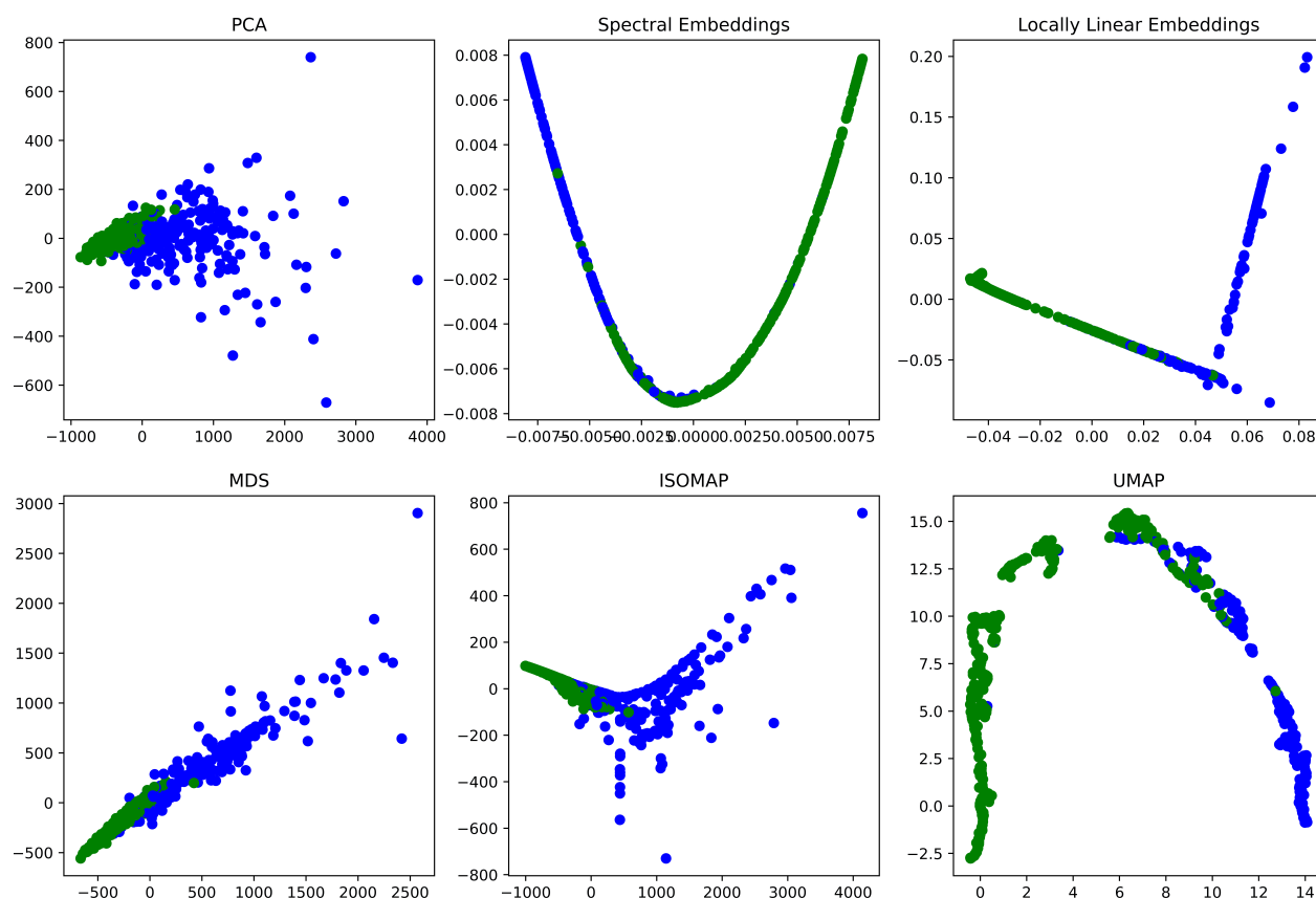
Рис. 9: Визуализация набора данных Breast Cancer после снижения размерности до 2 с использованием PCA, Spectral Embeddings, Locally Linear Embeddings, MDS, ISOMAP, UMAP.
