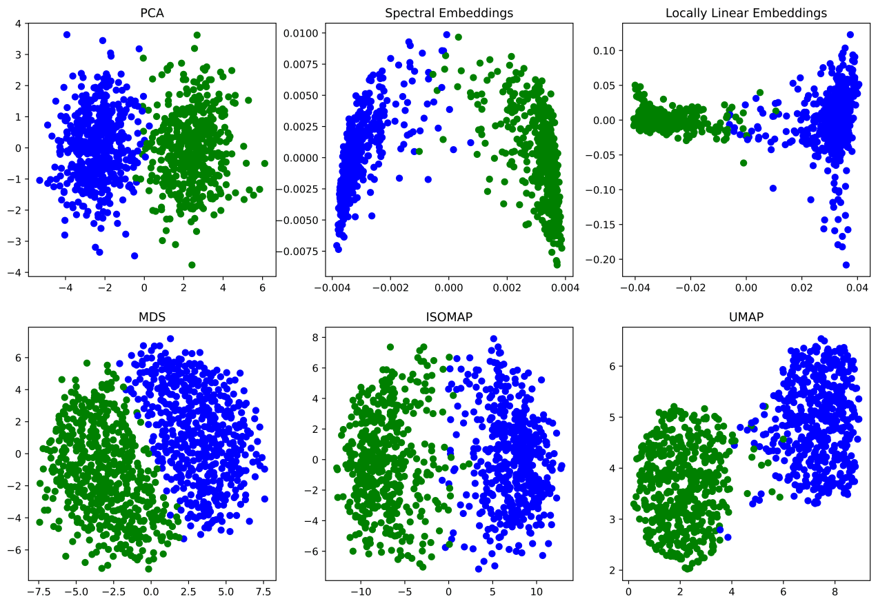
Рис. 2: Визуализация синтетических данных с параметром t = 0.4 после снижения размерности с 20 до 2 с использованием PCA, Spectral Embeddings, Locally Linear Embeddings, MDS, ISOMAP, UMAP.
