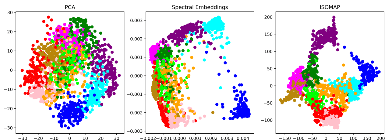
Рис. 11: Визуализация набора данных Digits после снижения размерности до 2 с использованием PCA, Spectral Embeddings, ISOMAP.
