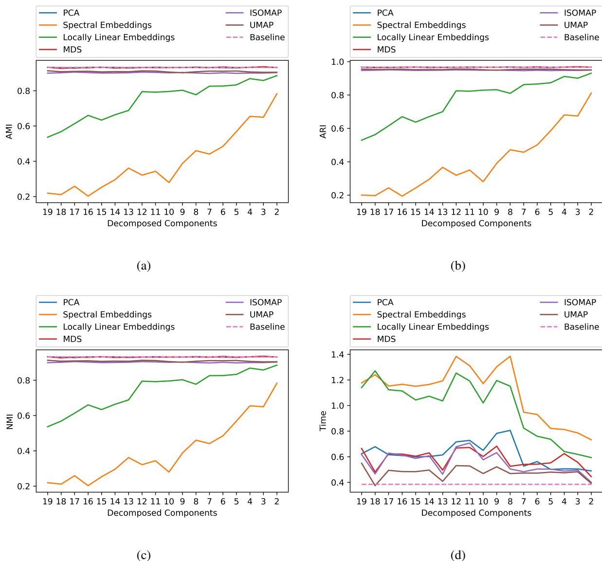
Рис. 3: Анализ влияния размерности данных при различных методах снижения размерности на кластеризацию синтетического набора данных с параметром t = 0.4 . Линия Baseline – результат работы алгоритма k -Means без предварительного снижения размерности. Результаты для (a) AMI; (b) ARI; (c) NMI, а также на время работы алгоритма (d).
