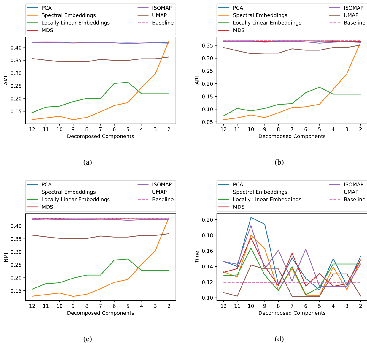
Рис. 12: Анализ влияния различных методов снижения размерности данных на кластеризацию набора данных Wine. Линия Baseline – результат работы алгоритма k -Means без предварительного снижения размерности. Результаты для (a) AMI; (b) ARI; (c) NMI, а также на время работы алгоритма (d).
