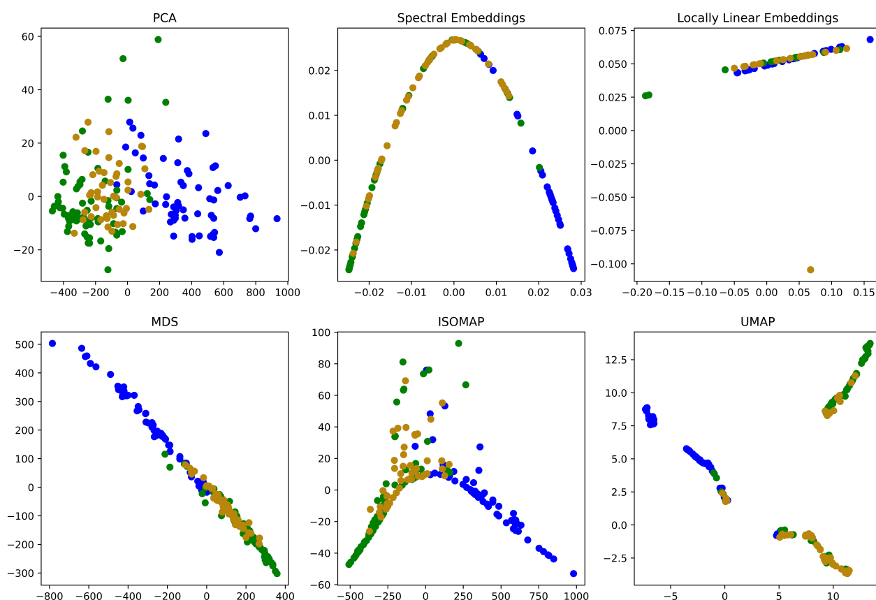
Рис. 13: Визуализация набора данных Wine после снижения размерности до 2 с использованием PCA, Spectral Embeddings, Locally Linear Embeddings, MDS, ISOMAP, UMAP.
