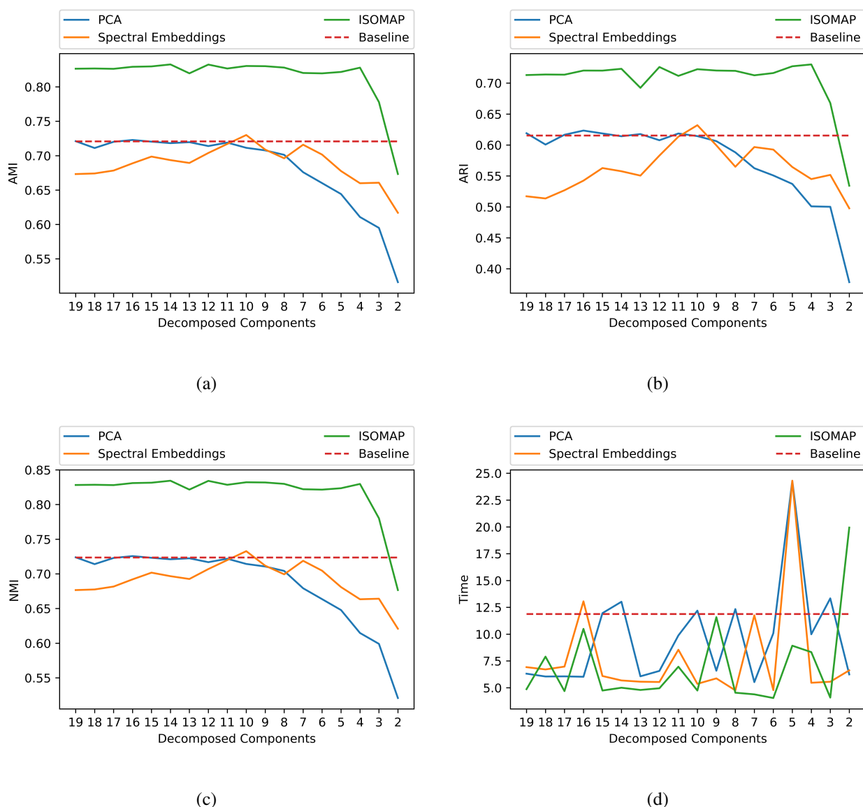
Рис. 5: Анализ влияния различных методов снижения размерности данных на кластеризацию набора данных Digits. Линия Baseline – результат работы алгоритма k -Means без предварительного снижения размерности. Результаты для (a) AMI; (b) ARI; (c) NMI, а также на время работы алгоритма (d).
