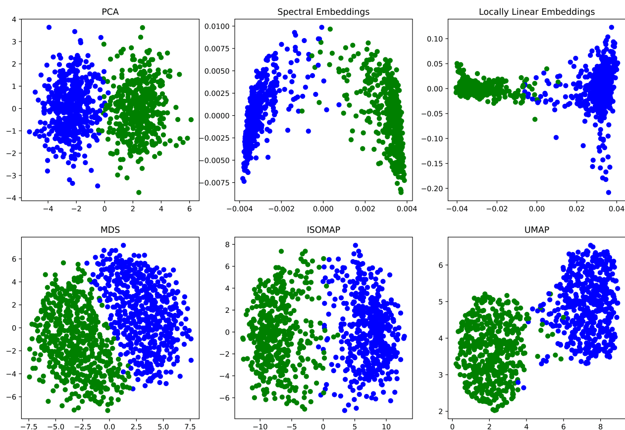
Рис. 2: Визуализация синтетических данных с параметром t = 0.4 после снижения размерности с 20 до 2 с использованием PCA, Spectral Embeddings, Locally Linear Embeddings, MDS, ISOMAP, UMAP.
