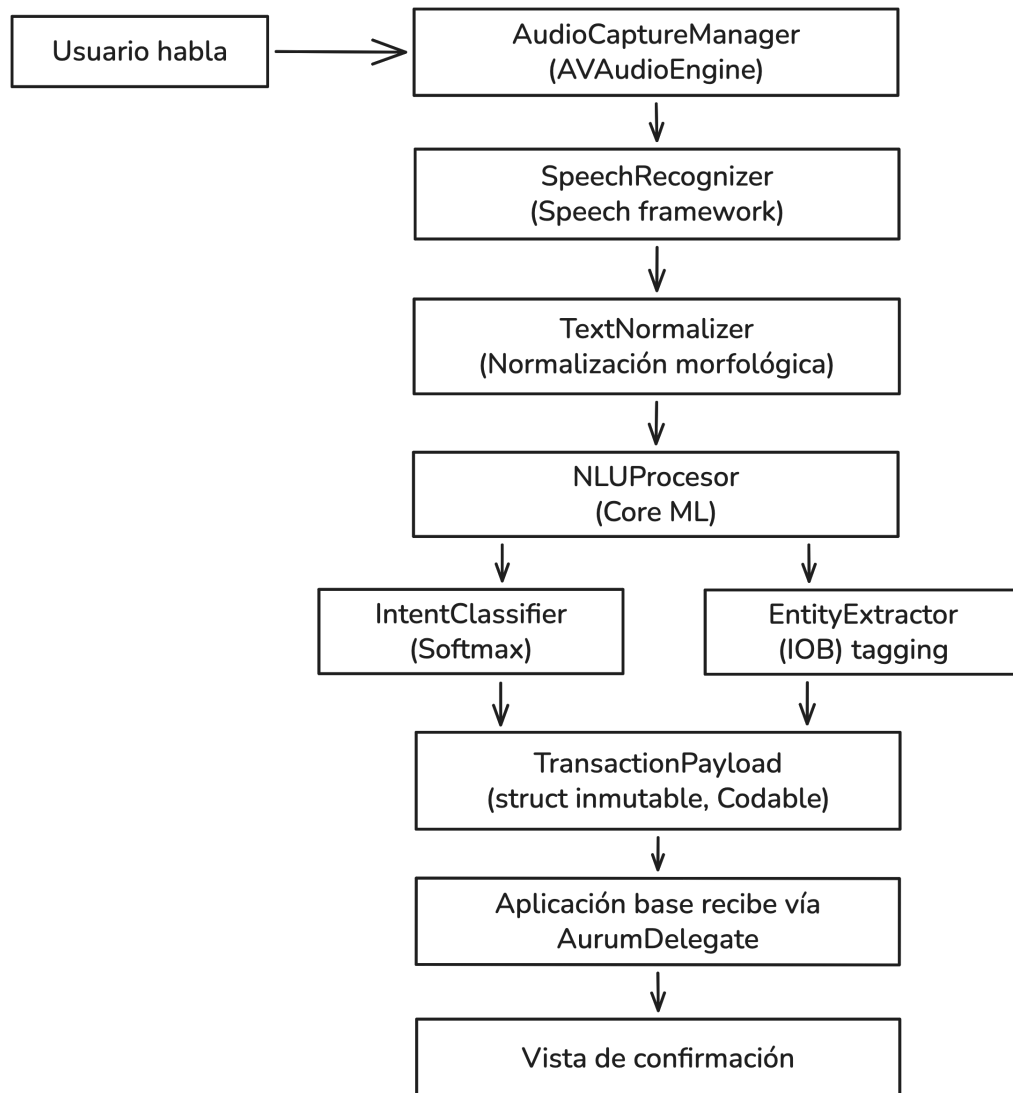
FIGURA 3.2. Flujo de pipeline.
