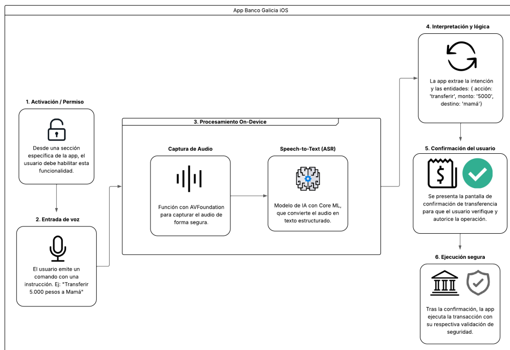
FIGURA 3.1. Diagrama de arquitectura de componentes.
