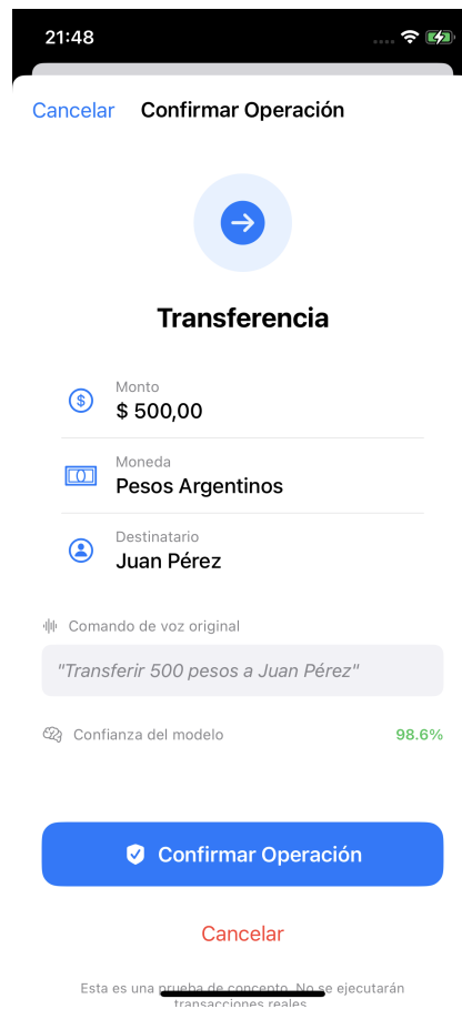
FIGURA 4.6. Pantalla de confirmación para una transferencia exitosa. Se muestra el monto ($ 500,00), la moneda (Pesos Argentinos), el destinatario (Juan Pérez), la transcripción original y la confianza del modelo (98.6 %).
