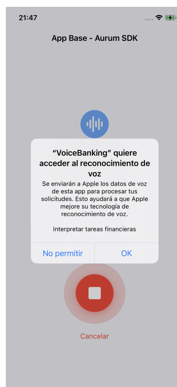
FIGURA 4.3. Solicitud de permiso de reconocimiento de voz (NSSpeech Recognition UsageDescription).
