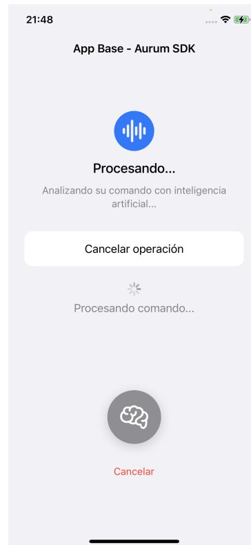
FIGURA 4.5. Estado processing: el botón se muestra gris con ícono de cerebro mientras los modelos Co- re ML ejecutan la inferencia.
