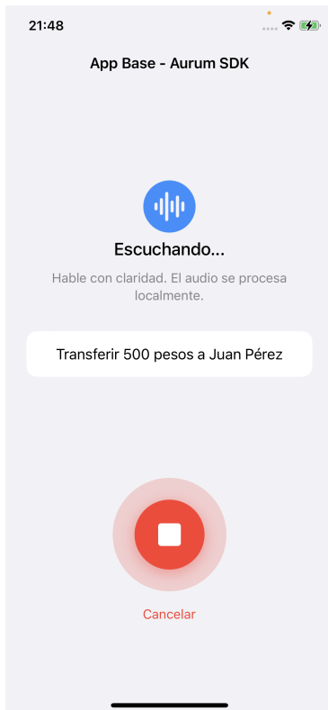
FIGURA 4.4. Estado listening: el botón mu- ta a rojo con animación de pulsación. La transcripción parcial se mues- tra en tiempo real.
