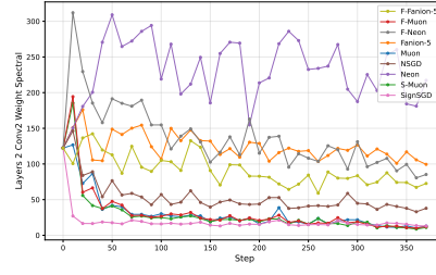
(d) Spectral norm of layer2.conv2
