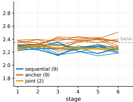
discriminability d'
