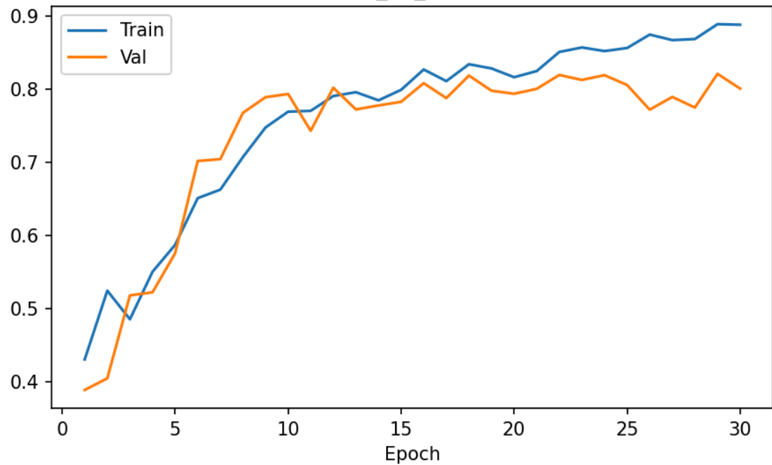
efficientnet_v2_s — Macro-F1
