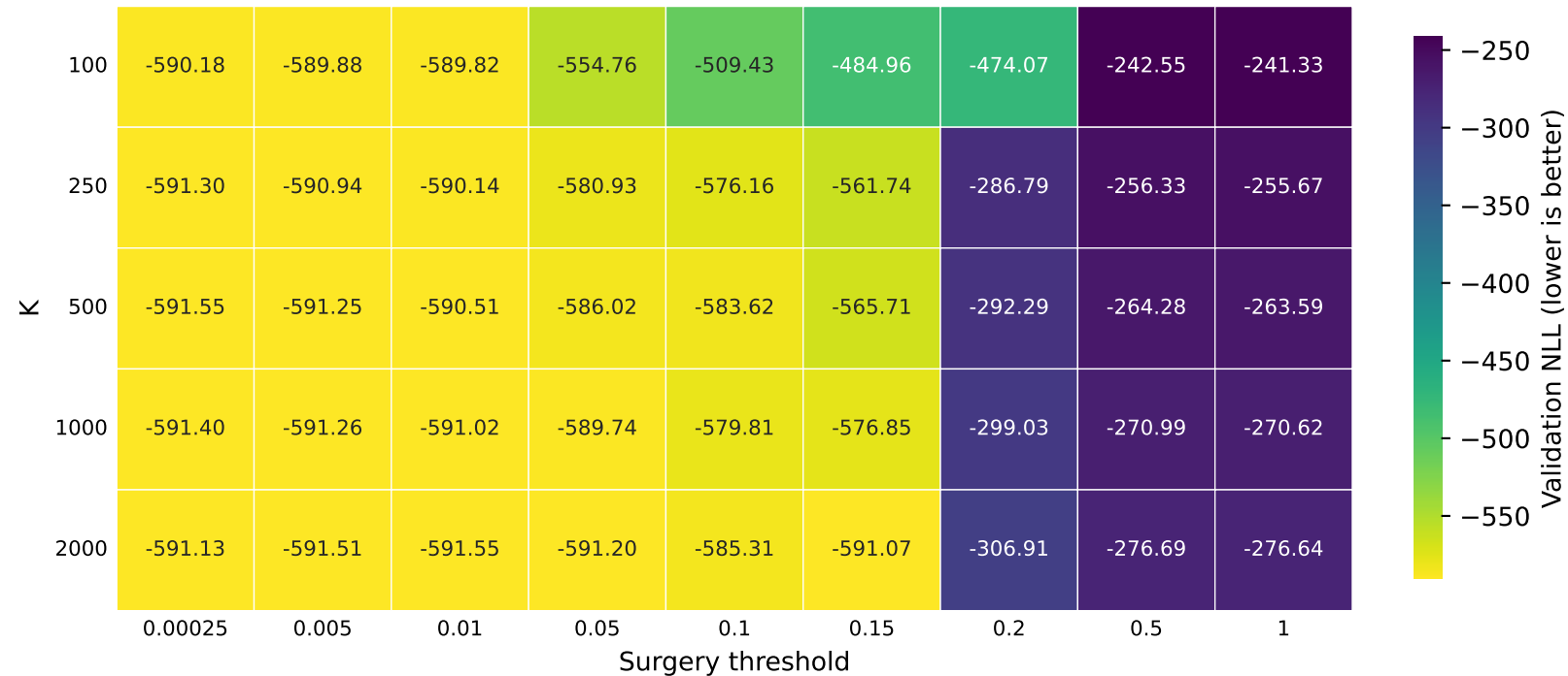
NLL (validation)
