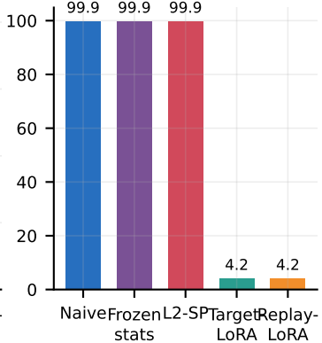
Trainable parameters
