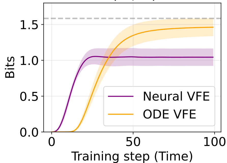
I(\mathcal{W}; \mathcal{A})
