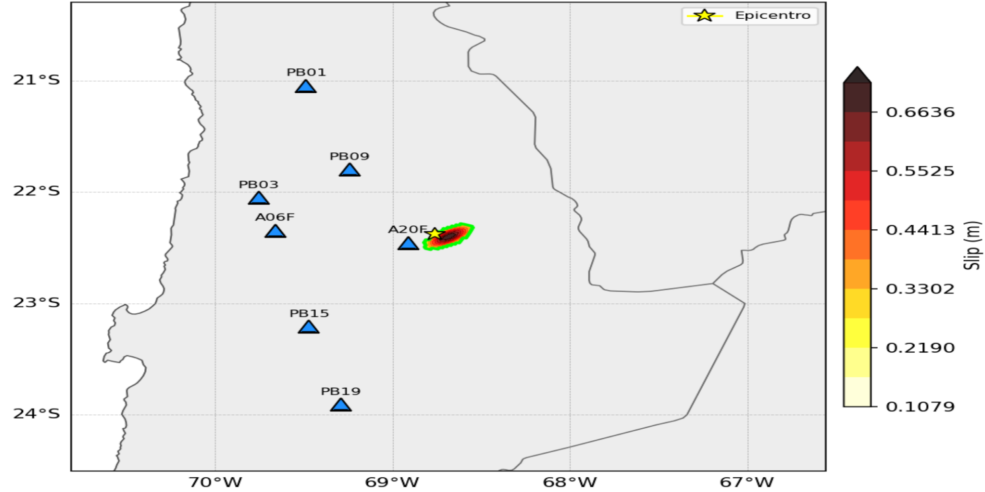
Cobertura azimutal — 7 estaciones gap máximo 225° (333°-558°)
