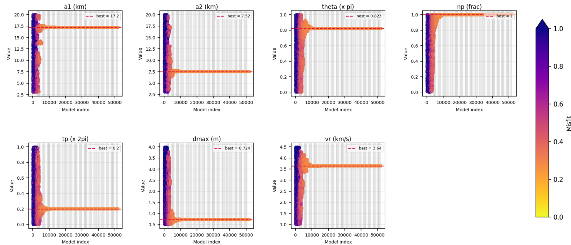
parameter convergence — NA search
