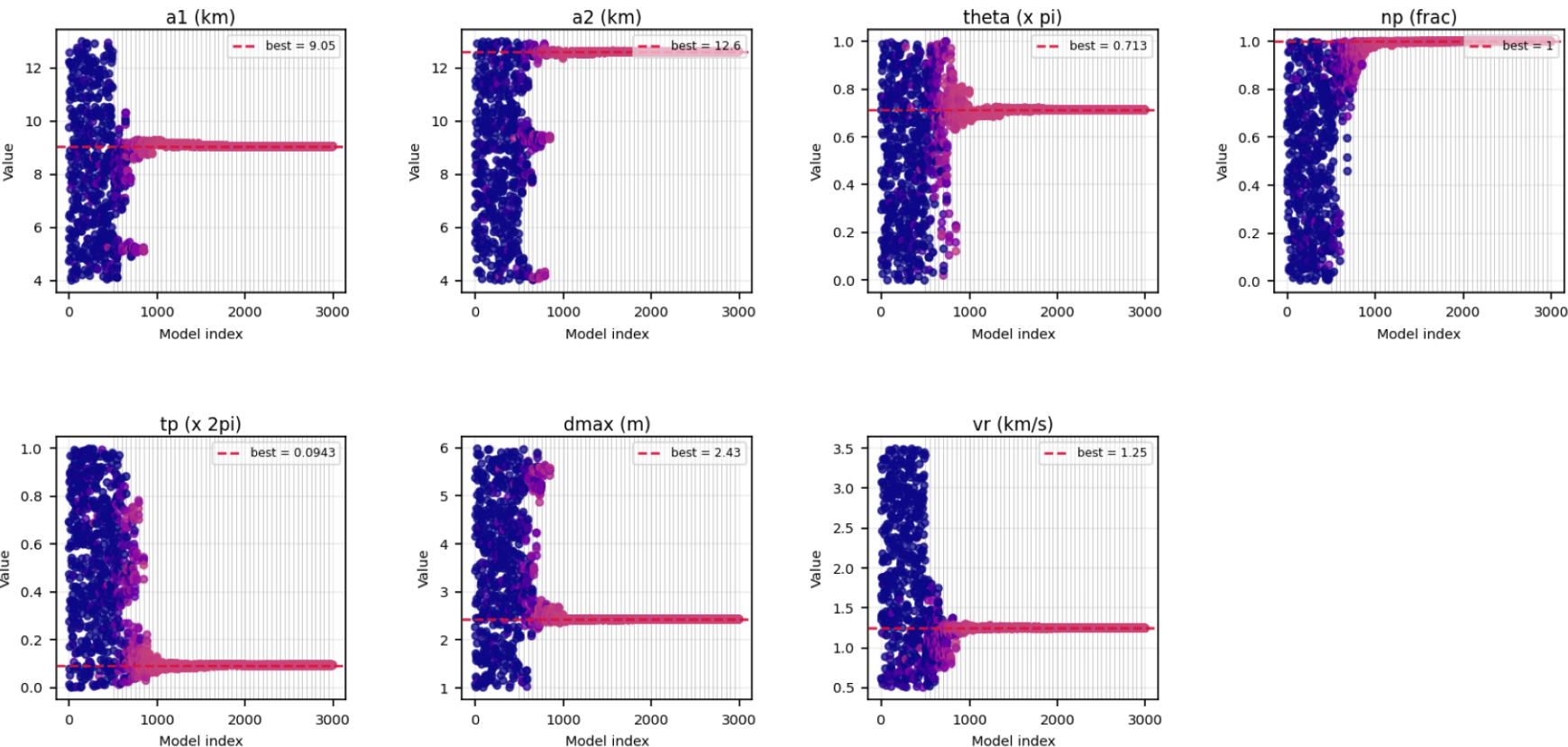
parameter convergence — Nelder-Mead
