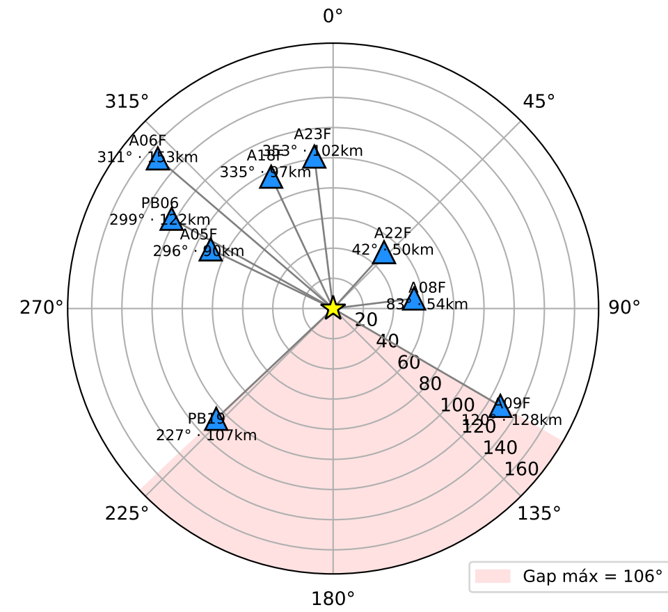
Cobertura azimutal — 9 estaciones gap máximo 106° (120°-227°)
