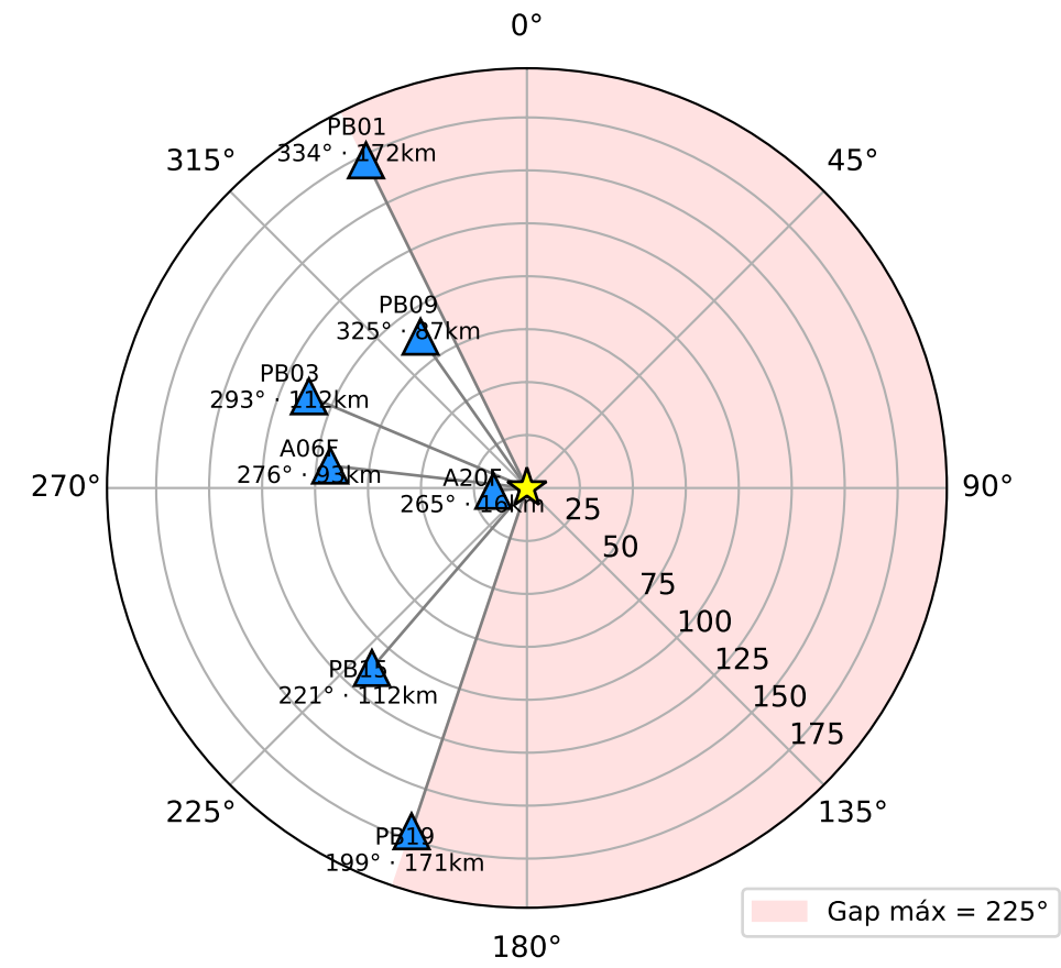
Cobertura azimuthal — 7 estaciones gap máximo 225° (334°-559°)
