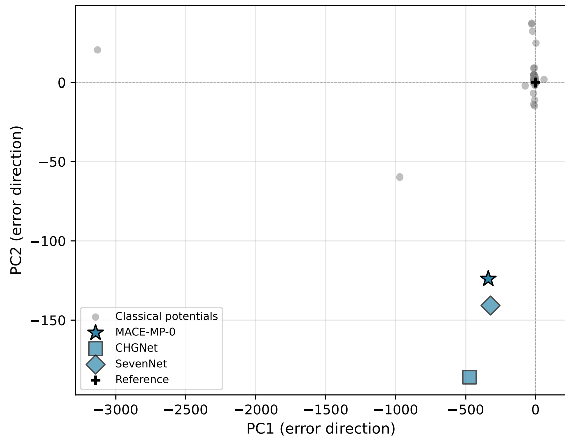
Cu (FCC)
