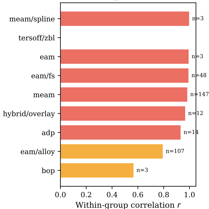
Per pair_style accuracy
