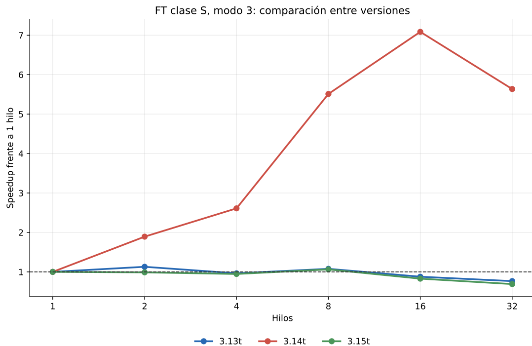
Figure 7.4: FT clase S, modo 3: speedup por versión de Python.
