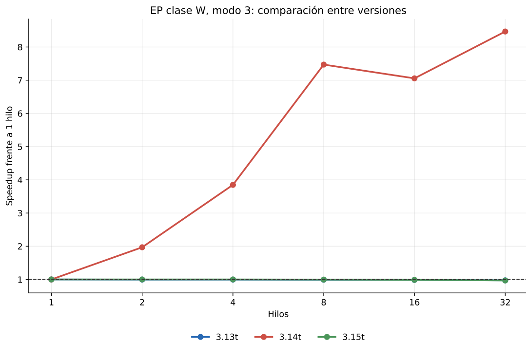
Figure 7.3: EP clase W, modo 3: speedup por versión de Python.
