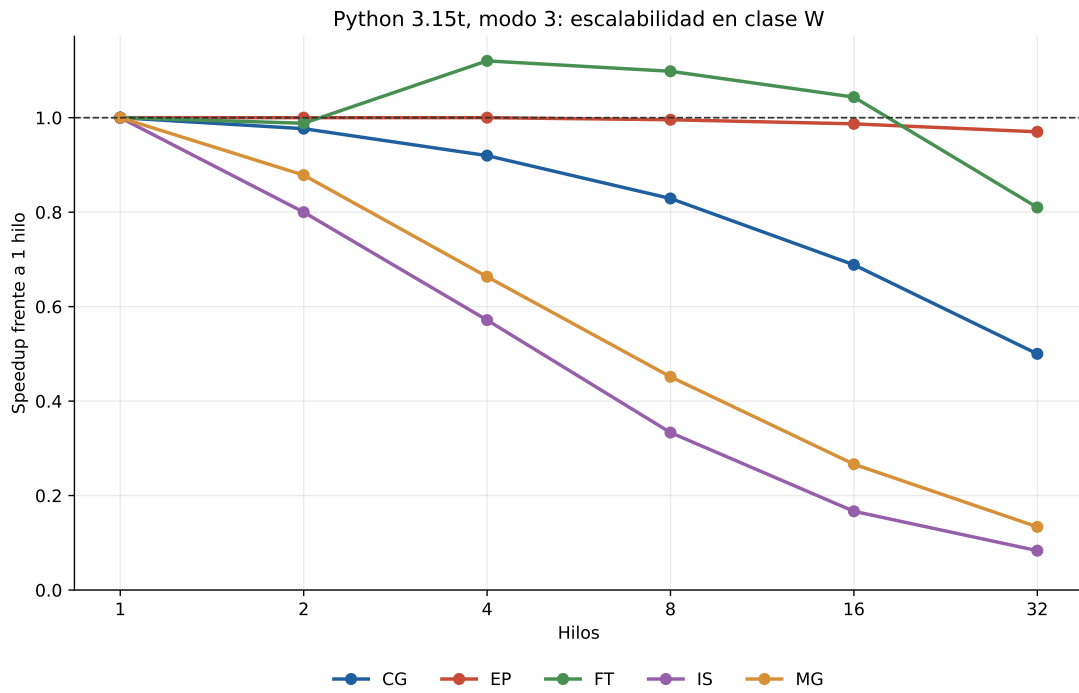
Figure 5.4: Speedup en clase W, modo 3, Python 3.15t.
