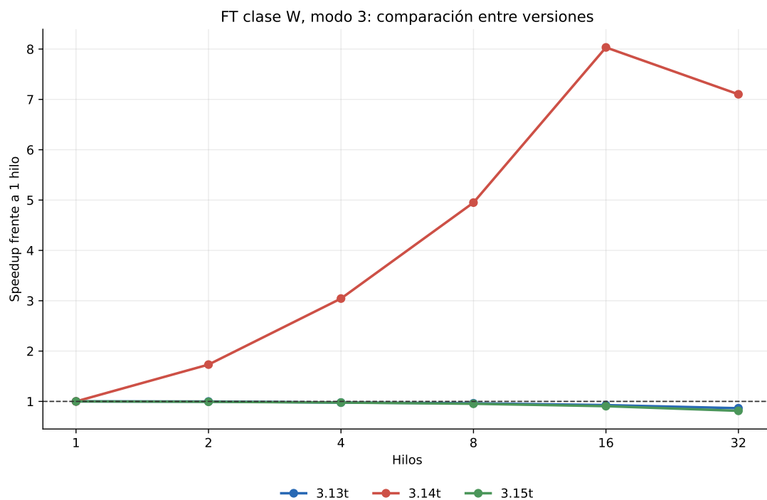
Figure 7.5: FT clase W, modo 3: speedup por versión de Python.
