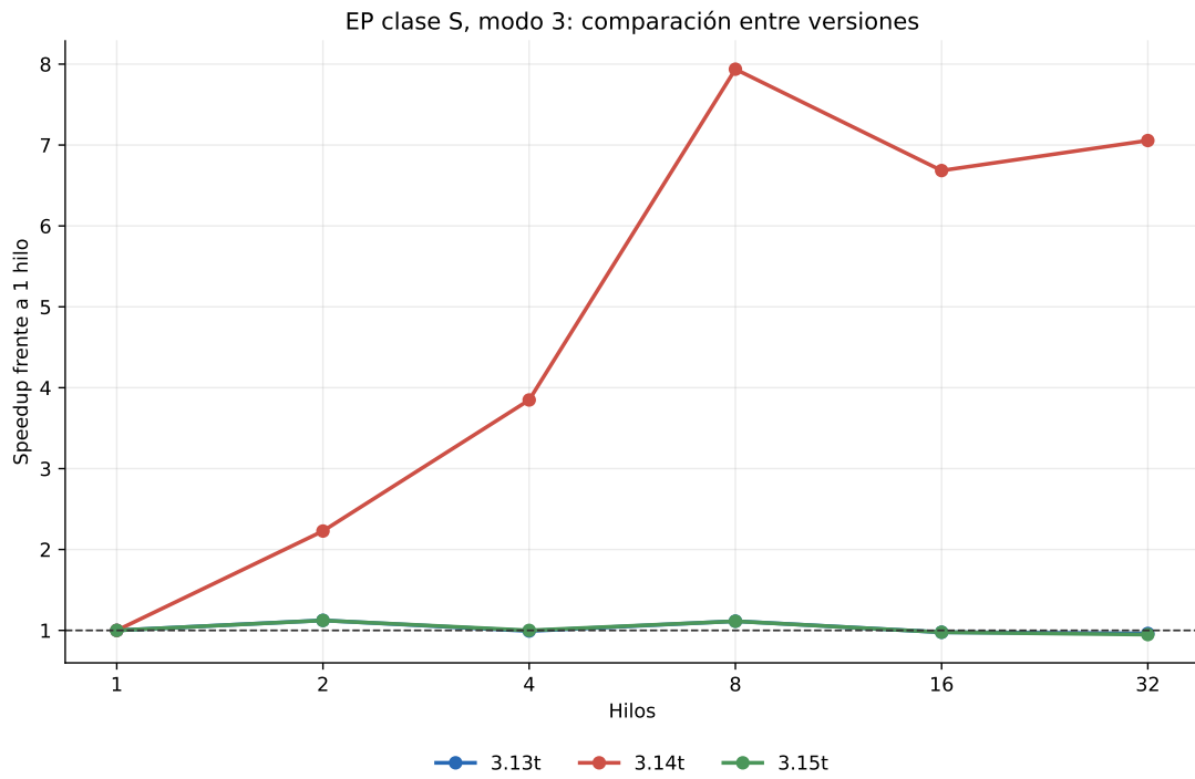
Figure 7.2: EP clase S, modo 3: speedup por versión de Python.
