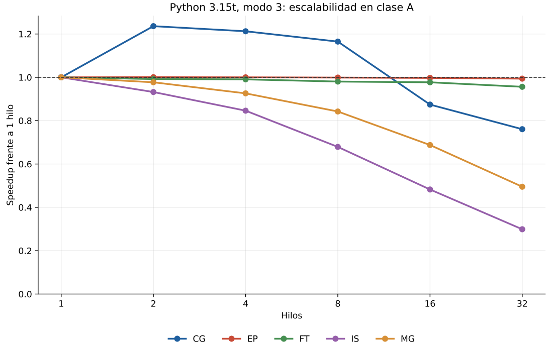
Figure 5.6: Speedup en clase A, modo 3, Python 3.15t.
