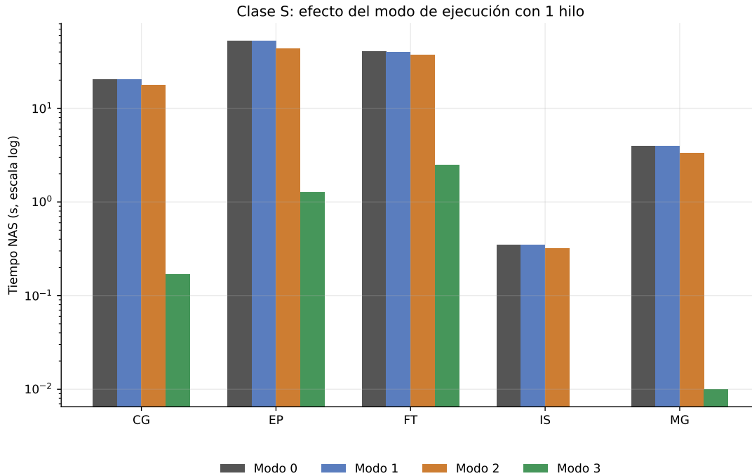
Figure 5.1: Tiempo NAS con un hilo en clase S para los cuatro modos de ejecución. El eje vertical usa escala logarítmica.
