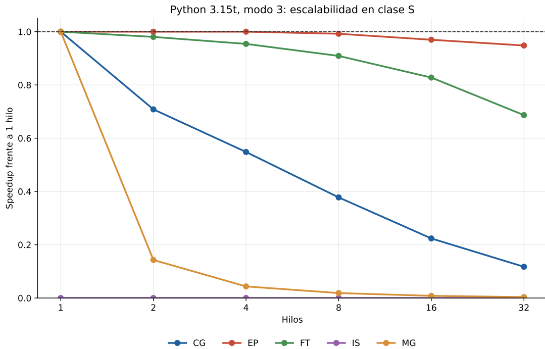
Figure 5.2: Speedup en clase S, modo 3, Python 3.15t. La línea discontinua marca el umbral de speedup 1.
