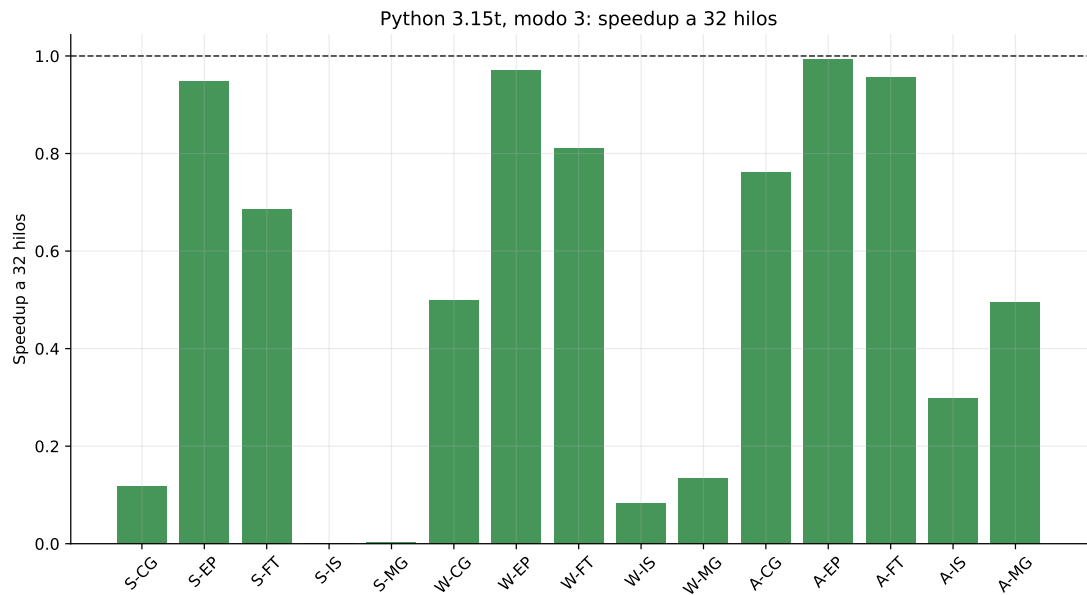
Figure 5.8: Speedup a 32 hilos en modo 3 para las clases S, W y A.
