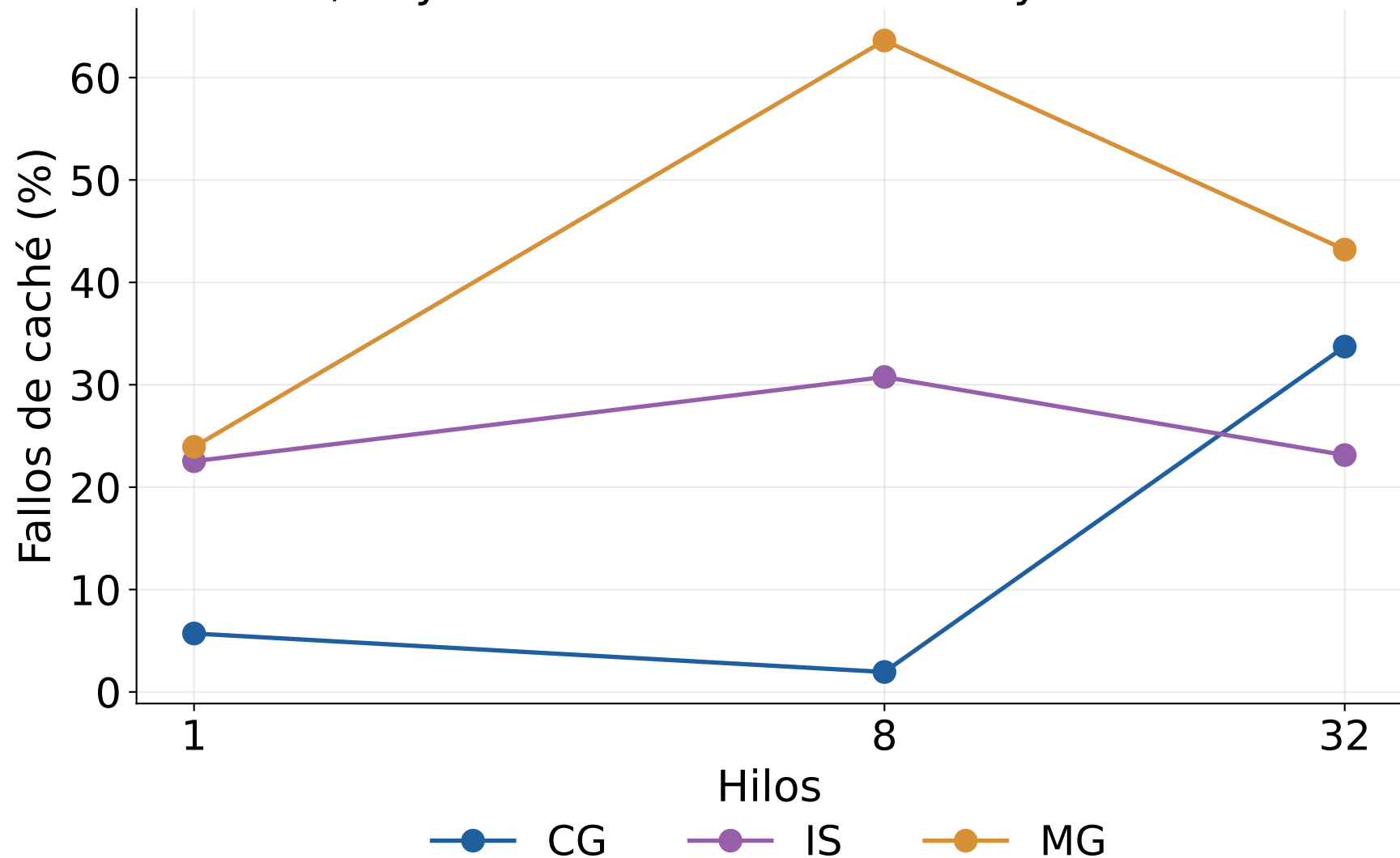
CG, IS y MG: fallos de caché en Python 3.13t
