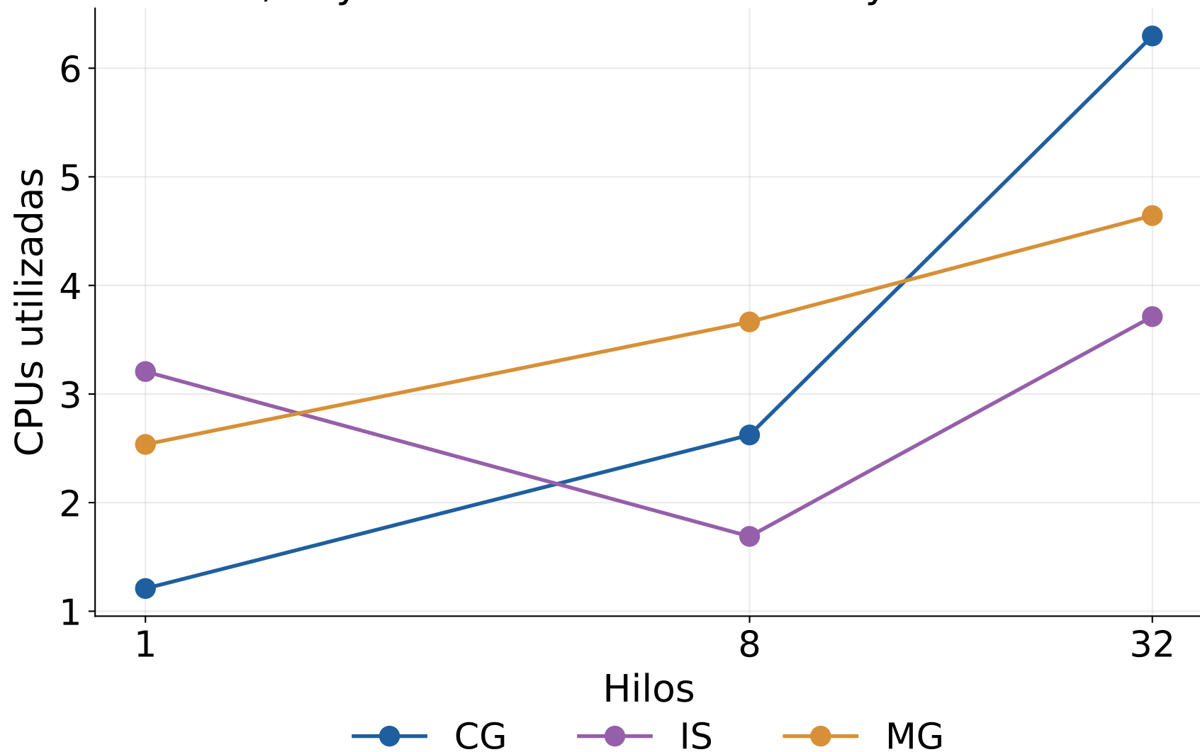
CG, IS y MG: CPUs utilizadas en Python 3.13t
