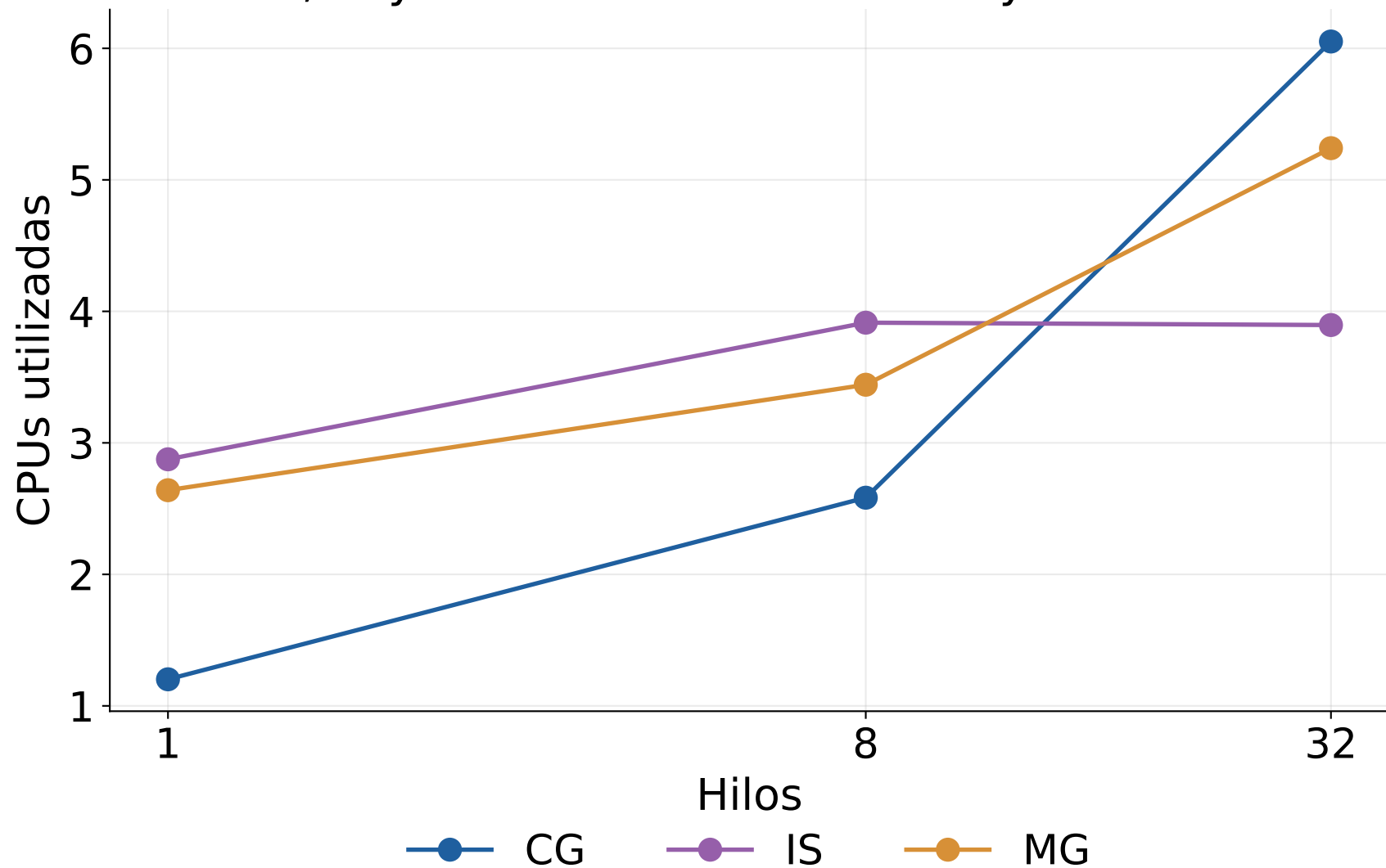
CG, IS y MG: CPUs utilizadas en Python 3.14t
