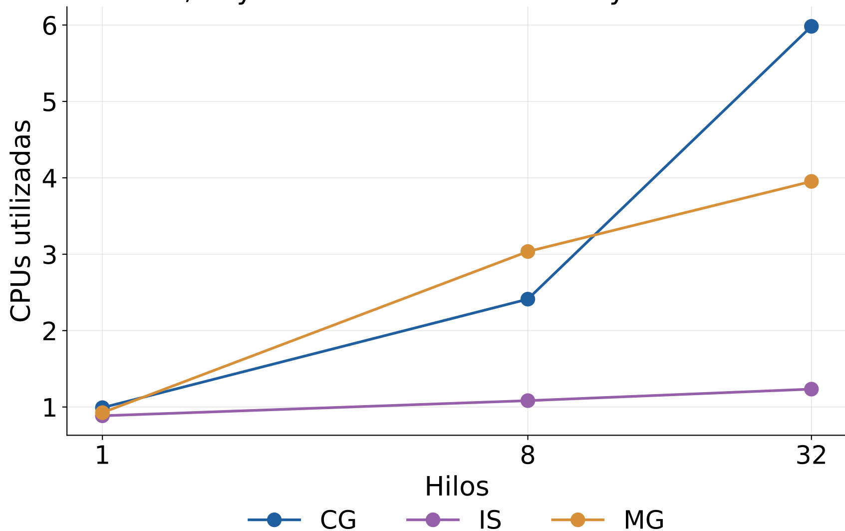
CG, IS y MG: CPUs utilizadas en Python 3.15t
