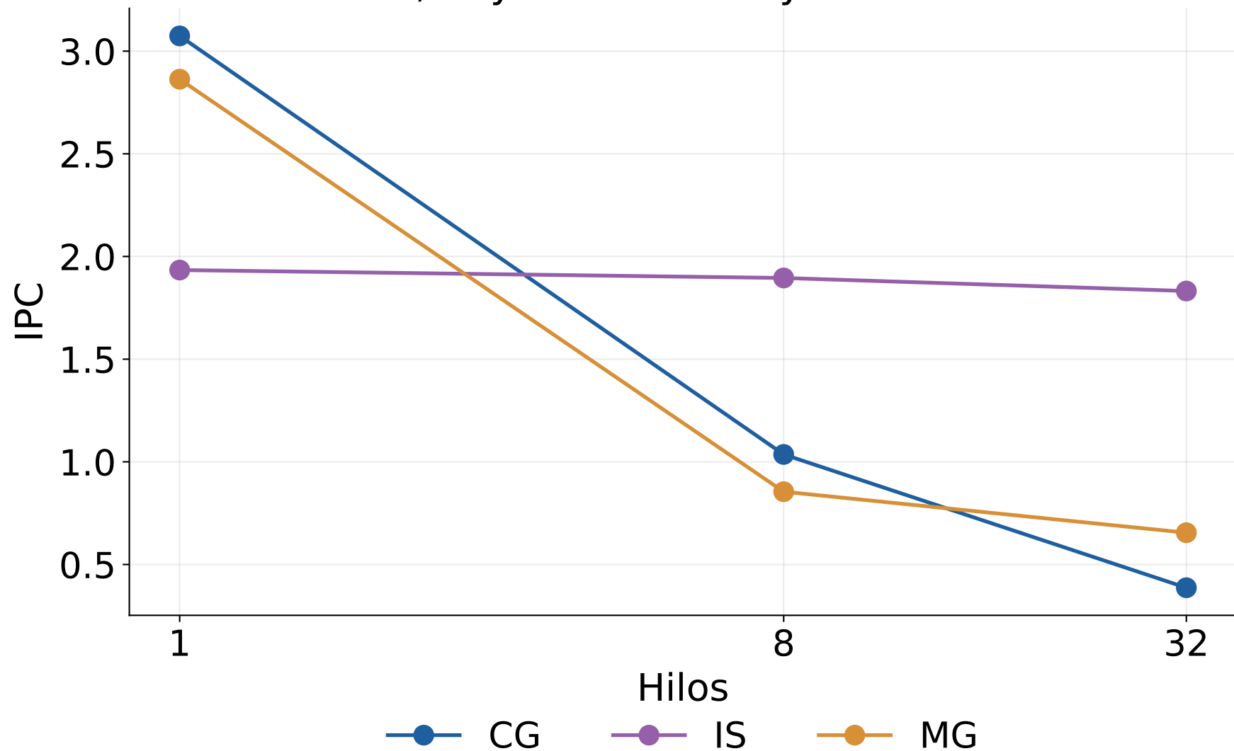
CG, IS y MG: IPC en Python 3.15t
