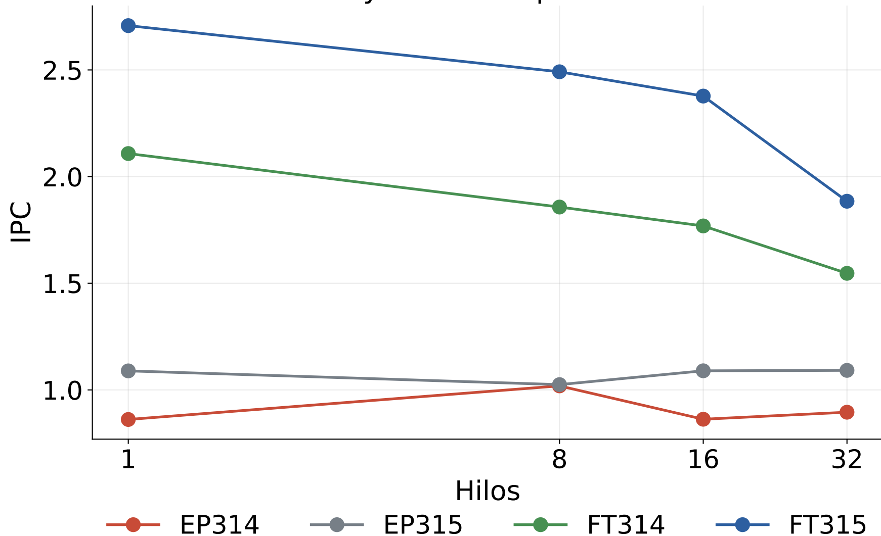
EP y FT: IPC en perf stat
