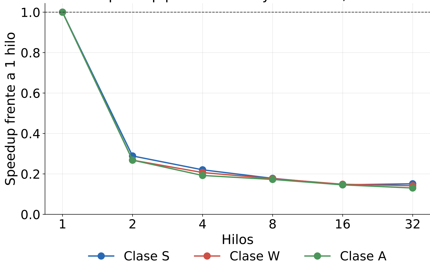
CG: speedup por clase en Python 3.15t, modo 3
