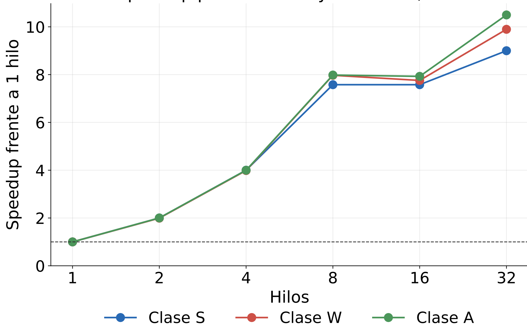
EP: speedup por clase en Python 3.15t, modo 3
