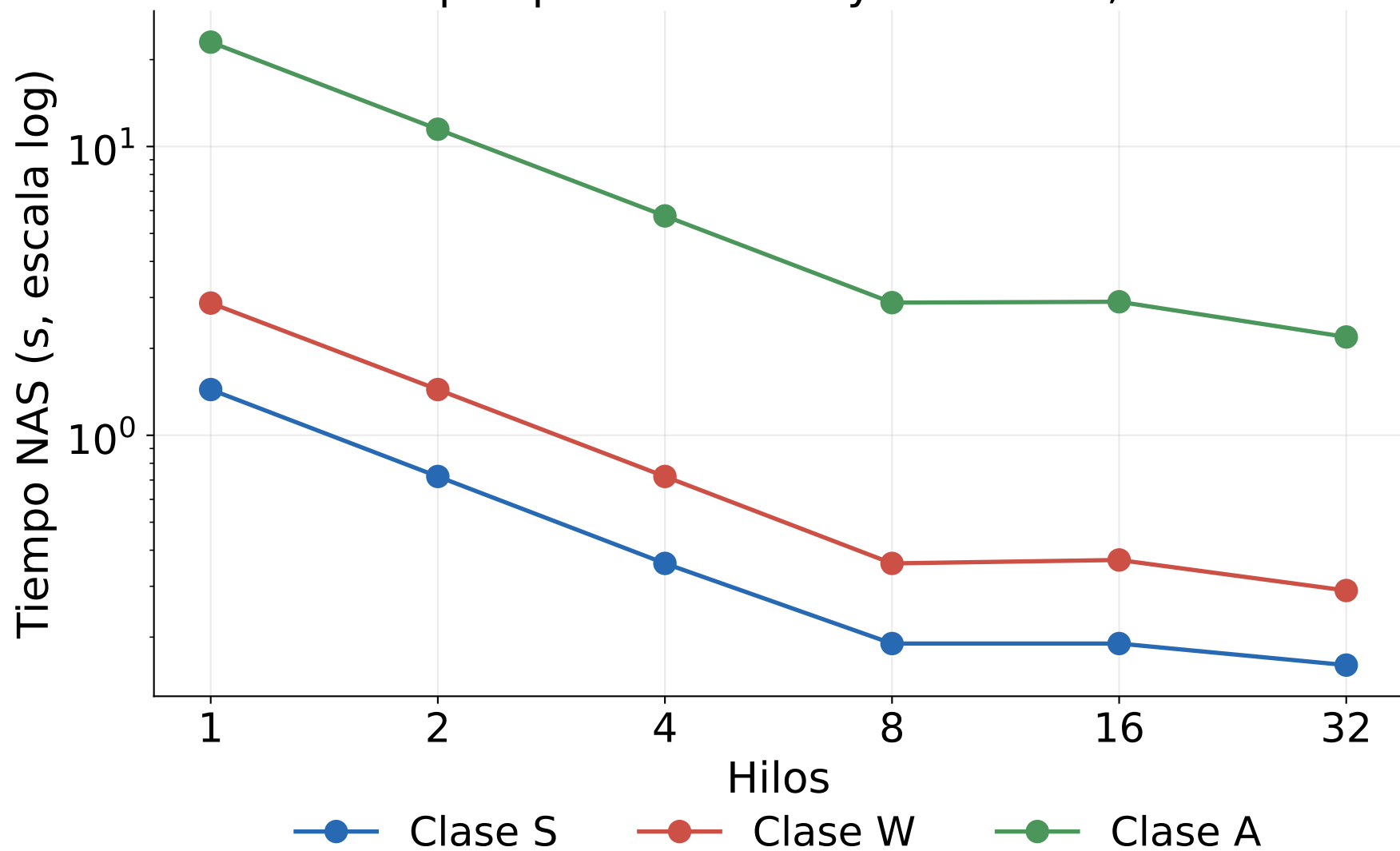
EP: tiempos por clase en Python 3.15t, modo 3
