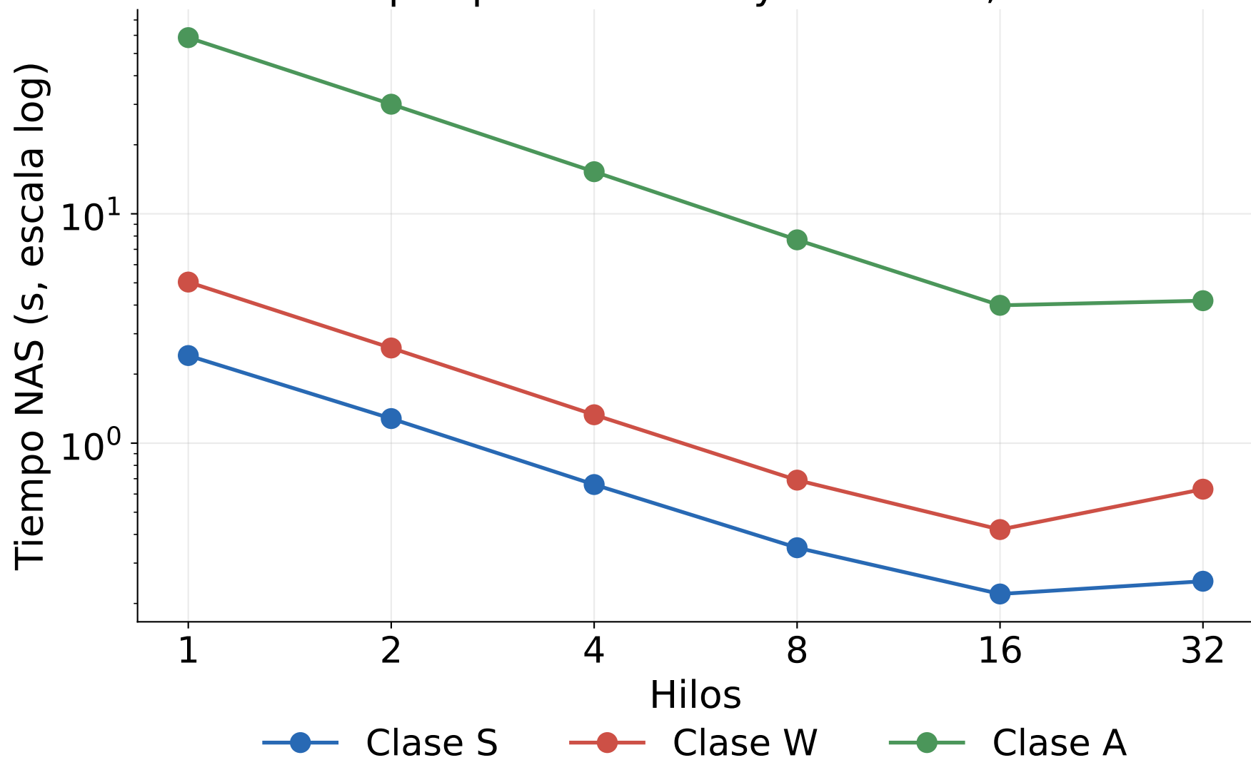
FT: tiempos por clase en Python 3.15t, modo 3
