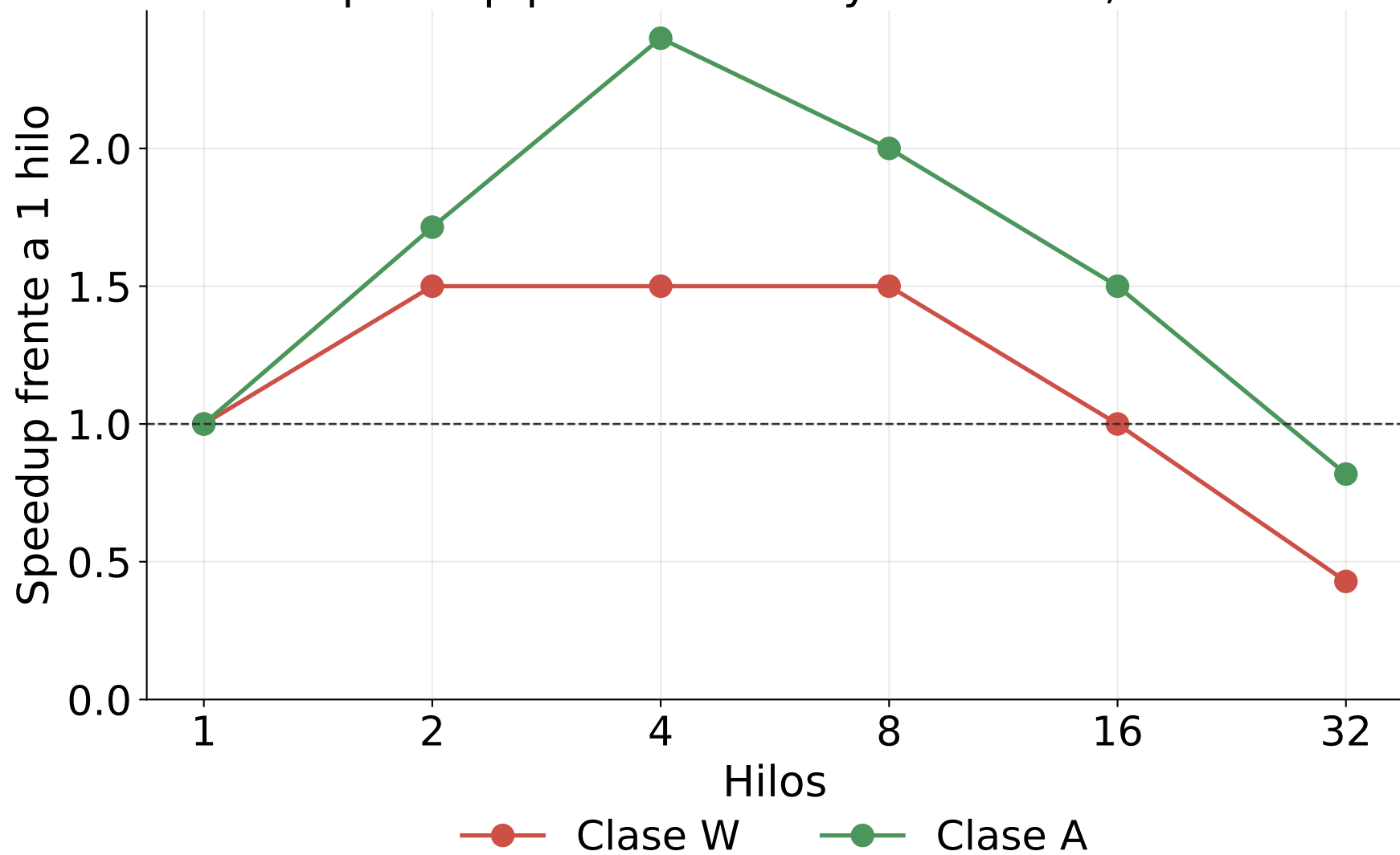
IS: speedup por clase en Python 3.15t, modo 3
