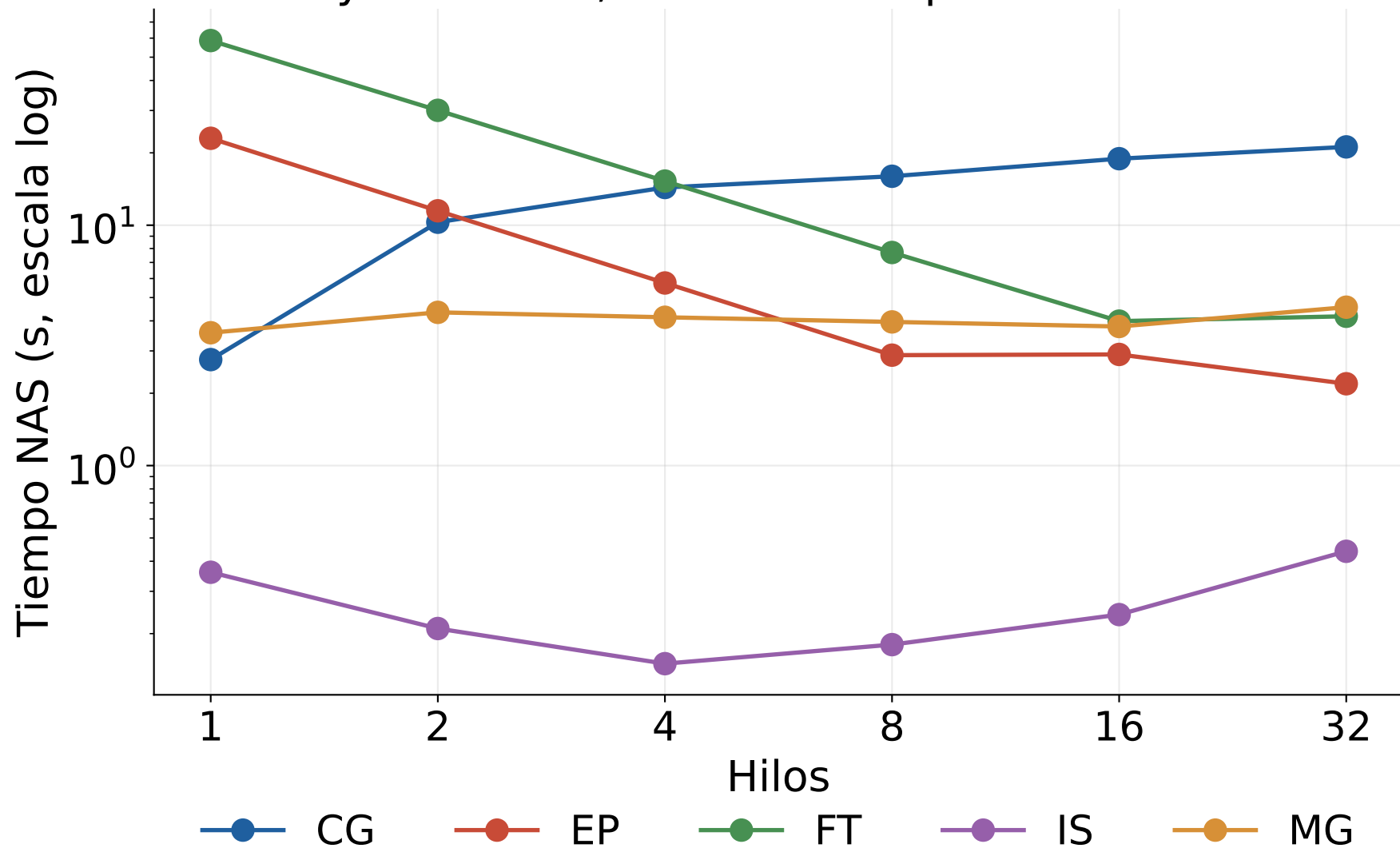
Python 3.15t, modo 3: tiempos en clase A
